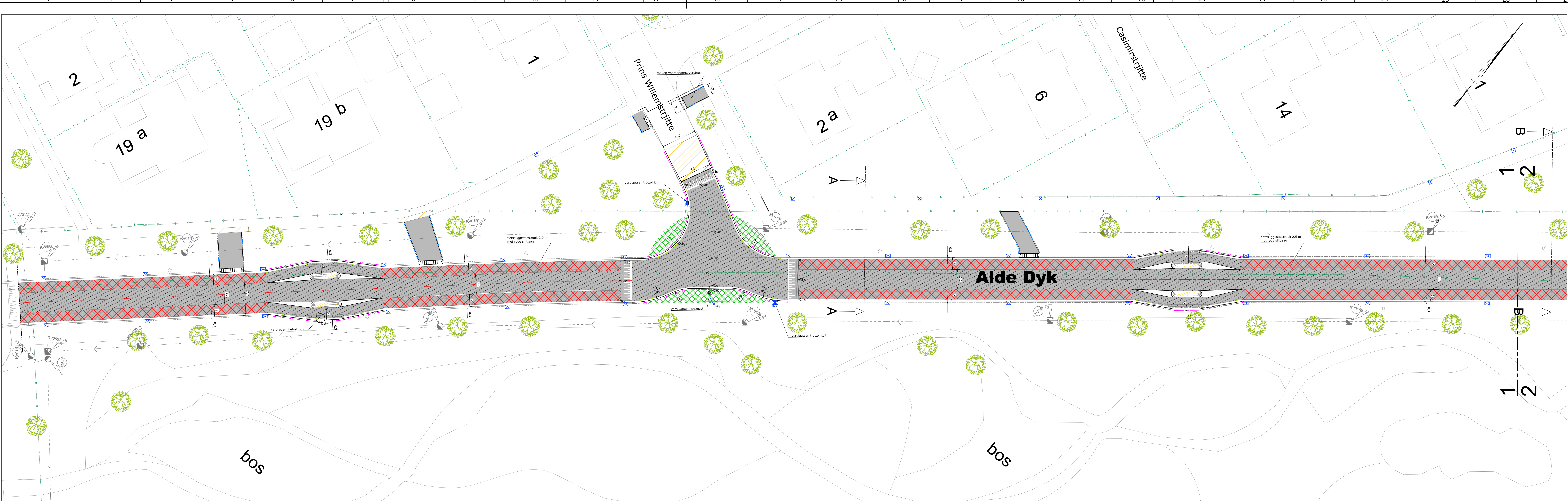
Situatie herinrichting rijbaan Alde Dyk Centrum Fase II Kootstertille
