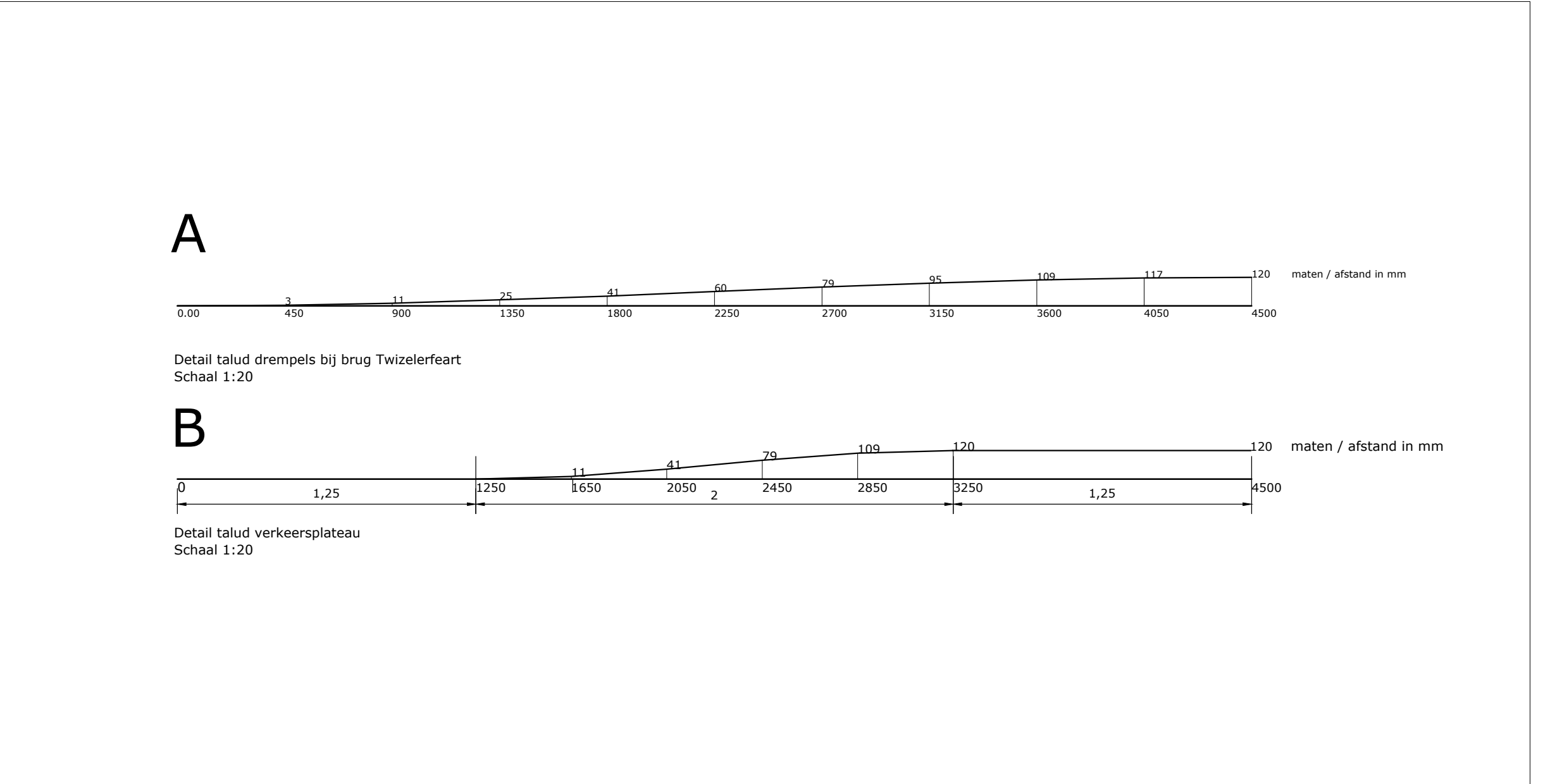
Langteprofiel talud verkeersplateau / drempels (schaal 1:20)
