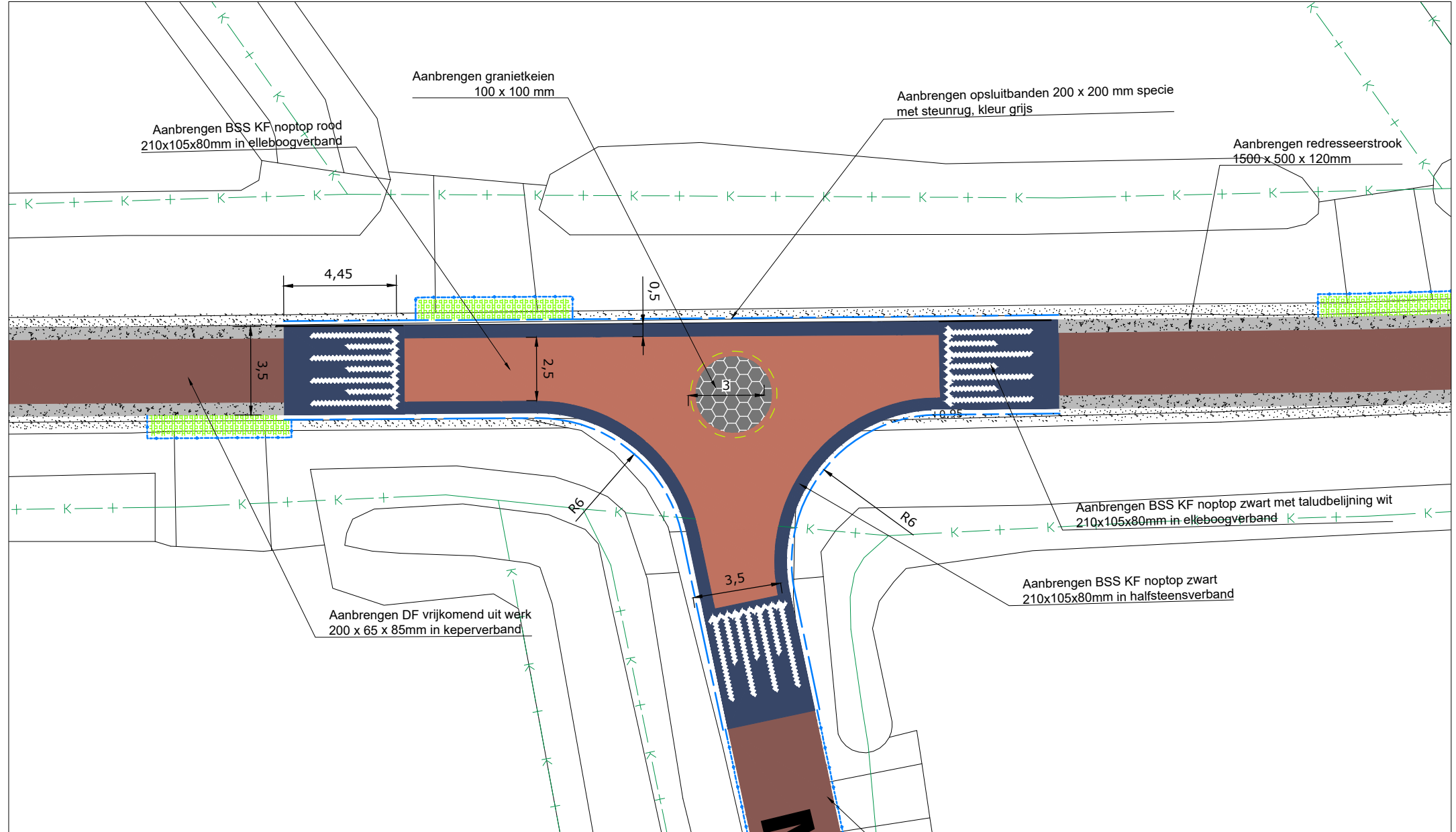
Detail 2 (schaal 1:200)
