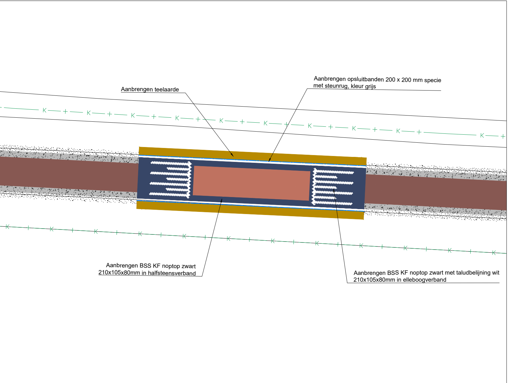
Detail 4 (schaal 1:200)
