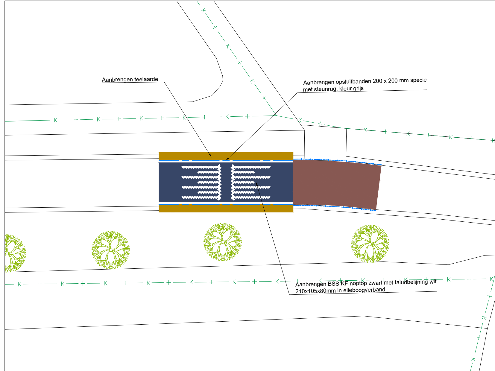
Detail 1 (schaal 1:200)
