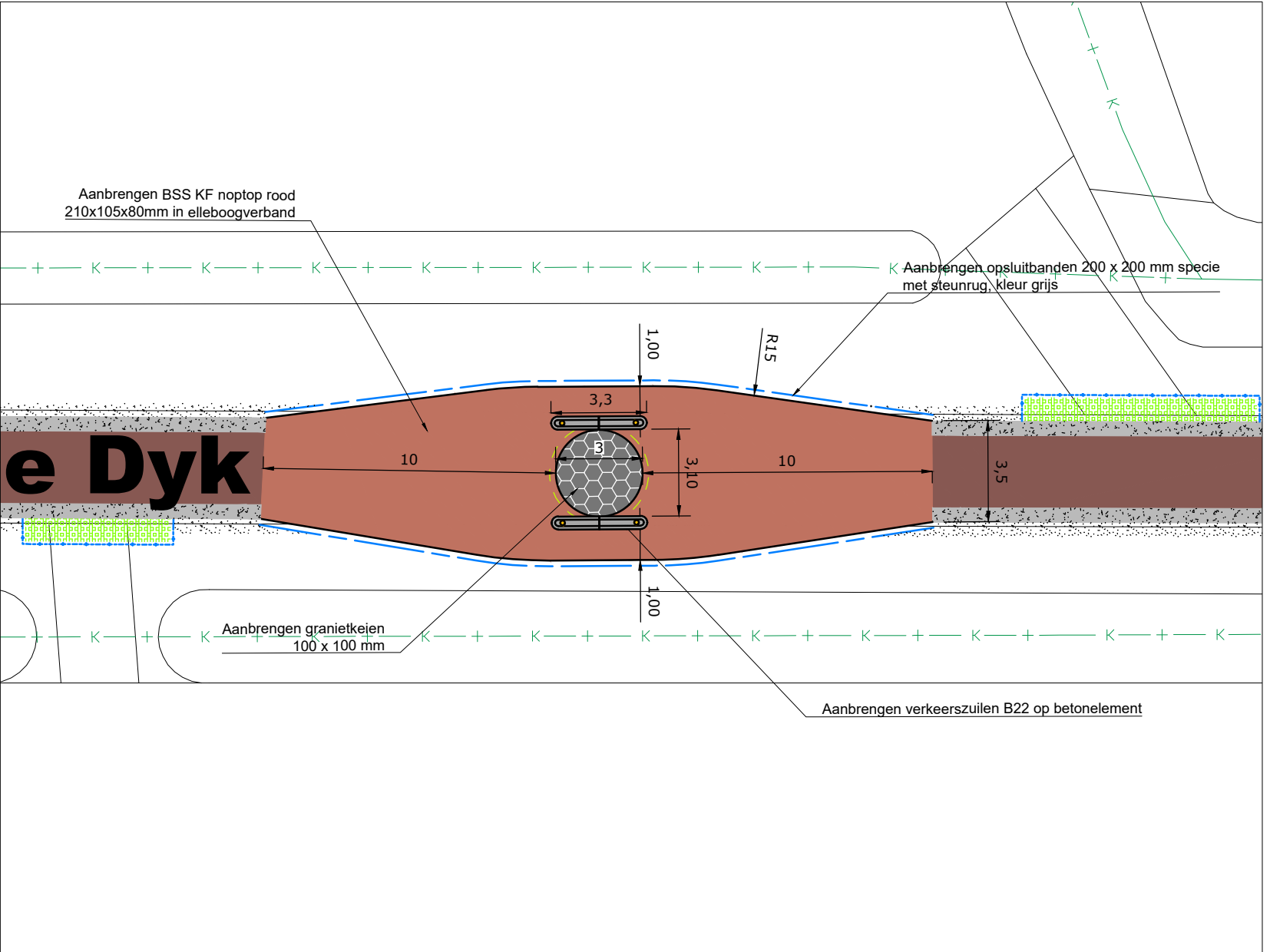
Detail 3 (schaal 1:200)
