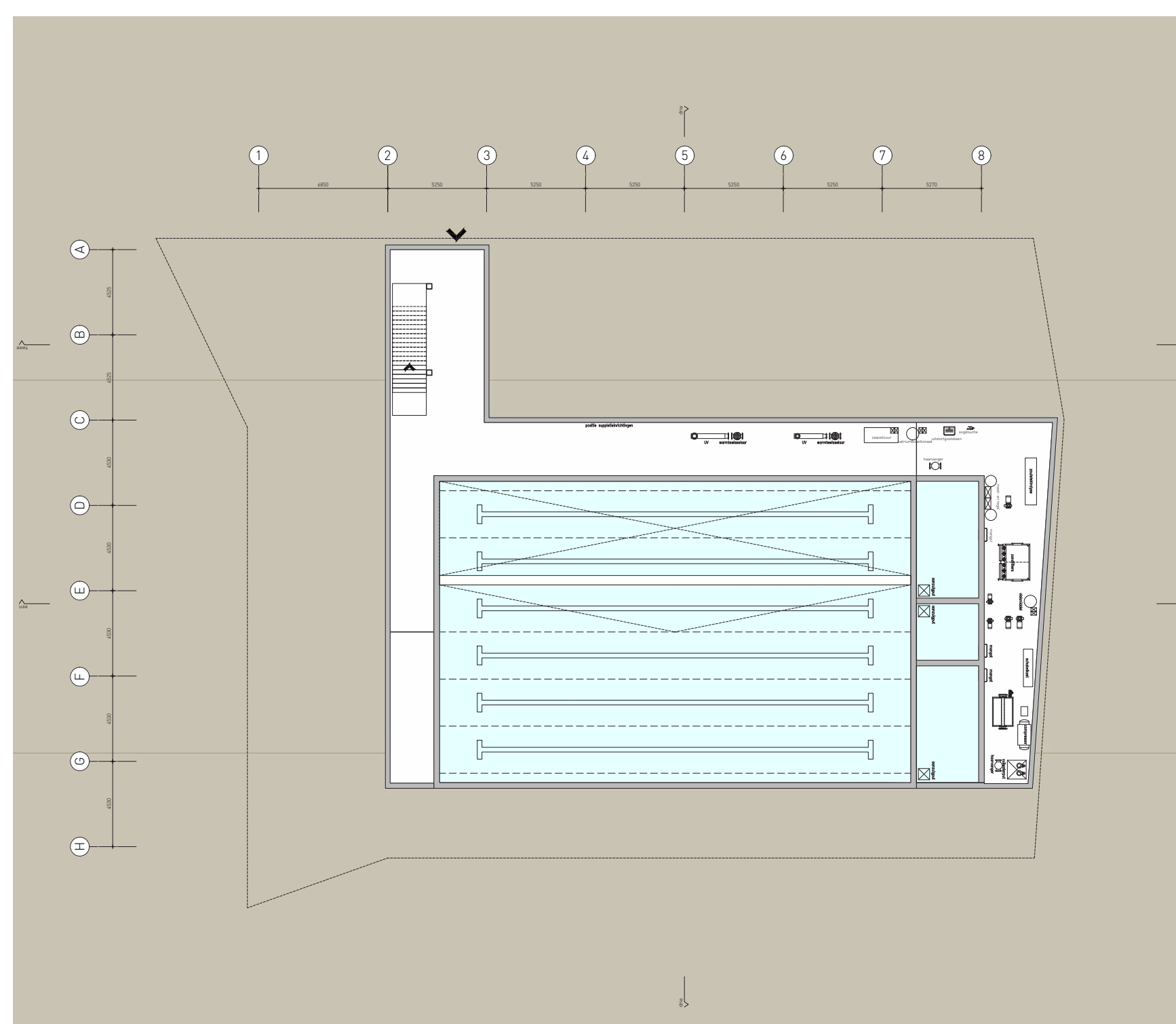
Kelder
