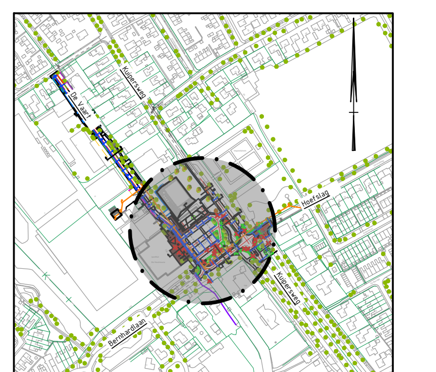
Overzicht Buitenpost 1:5000
