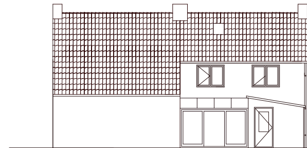
Achtergevel
