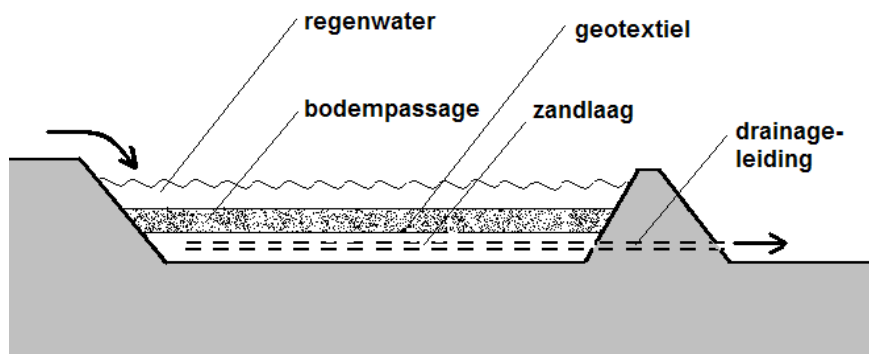
Opbouw van een bodempassage
