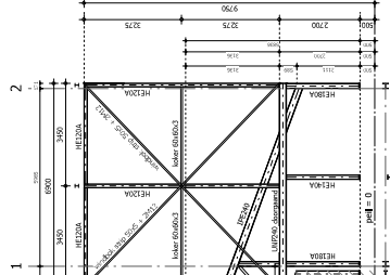
CONSTRUCTIE AS J
