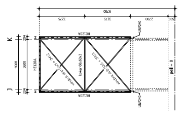
CONSTRUCTIE LW T.P.V. AS J - K
