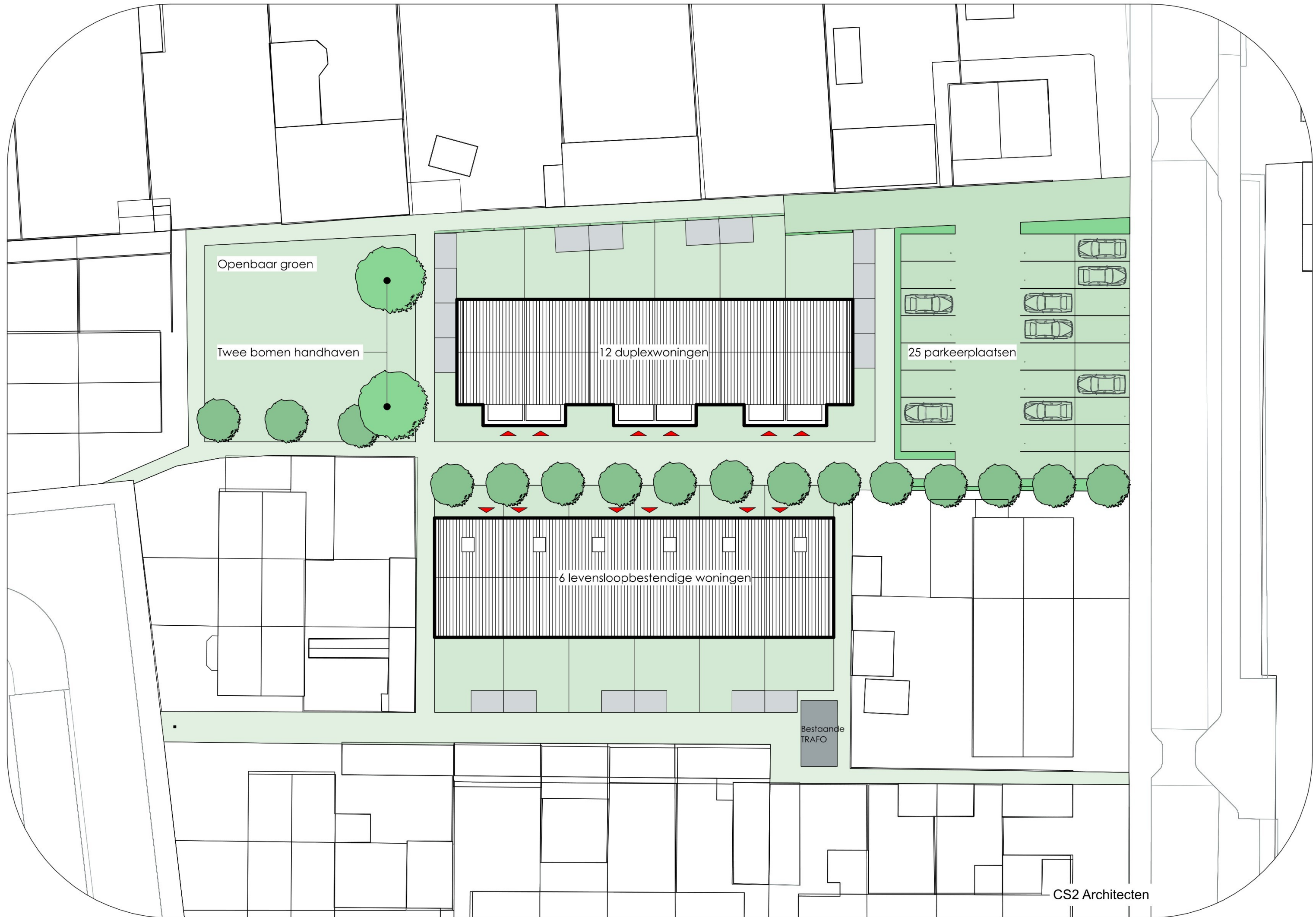
PLAN OVERZICHT schaal 1:300
