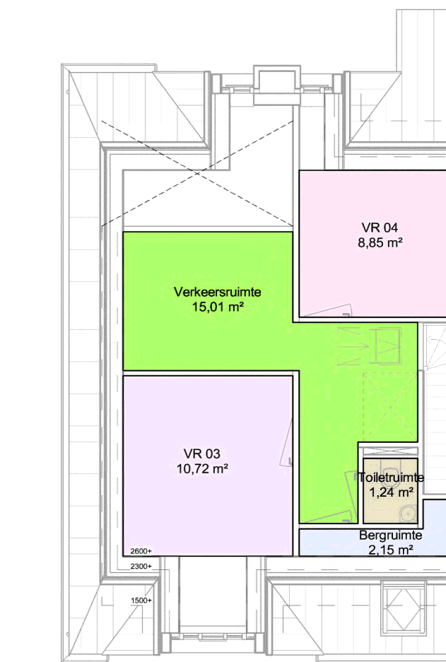
Eerste verdieping Ruimten
