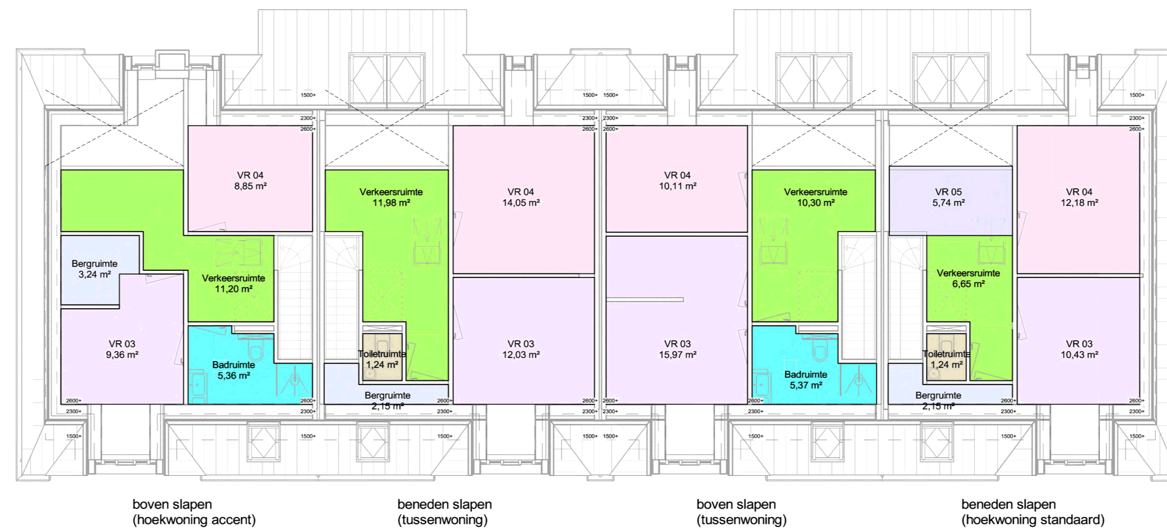
Eerste verdieping Ruimten
