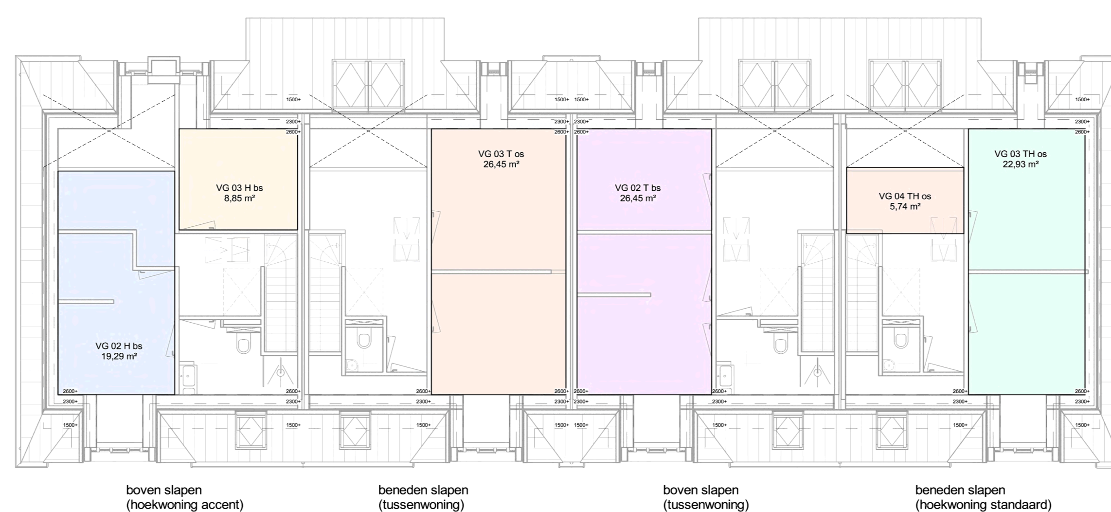
Eerste verdieping VG
