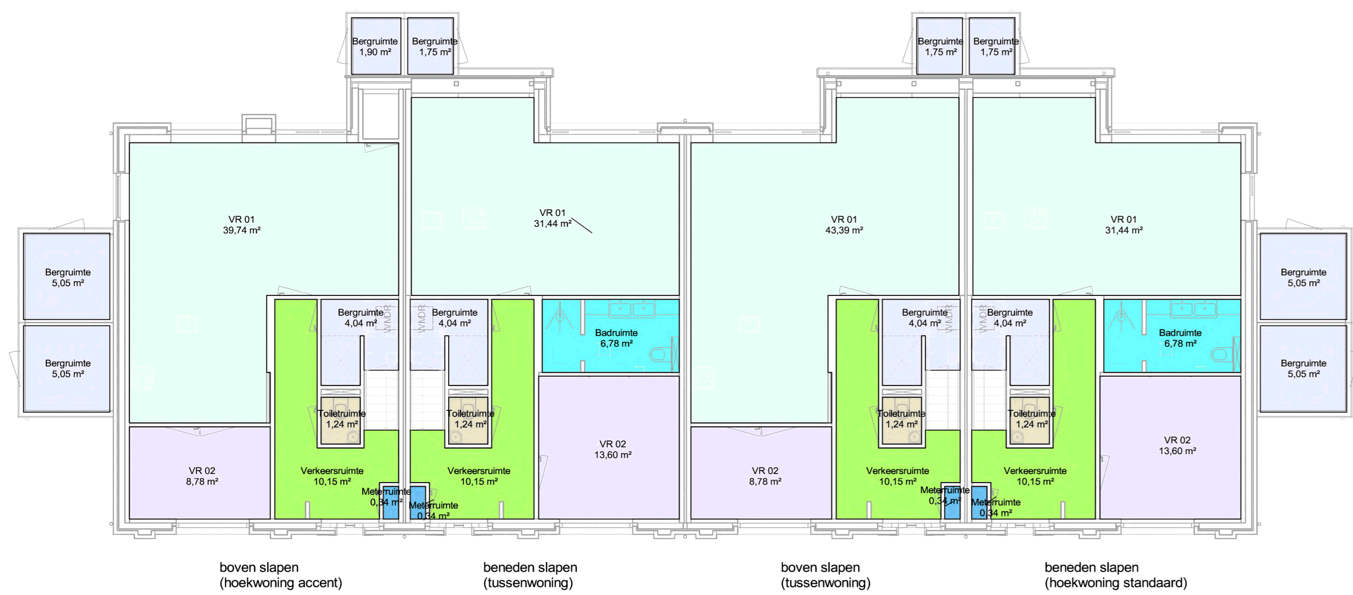
Begane grond Ruimten
