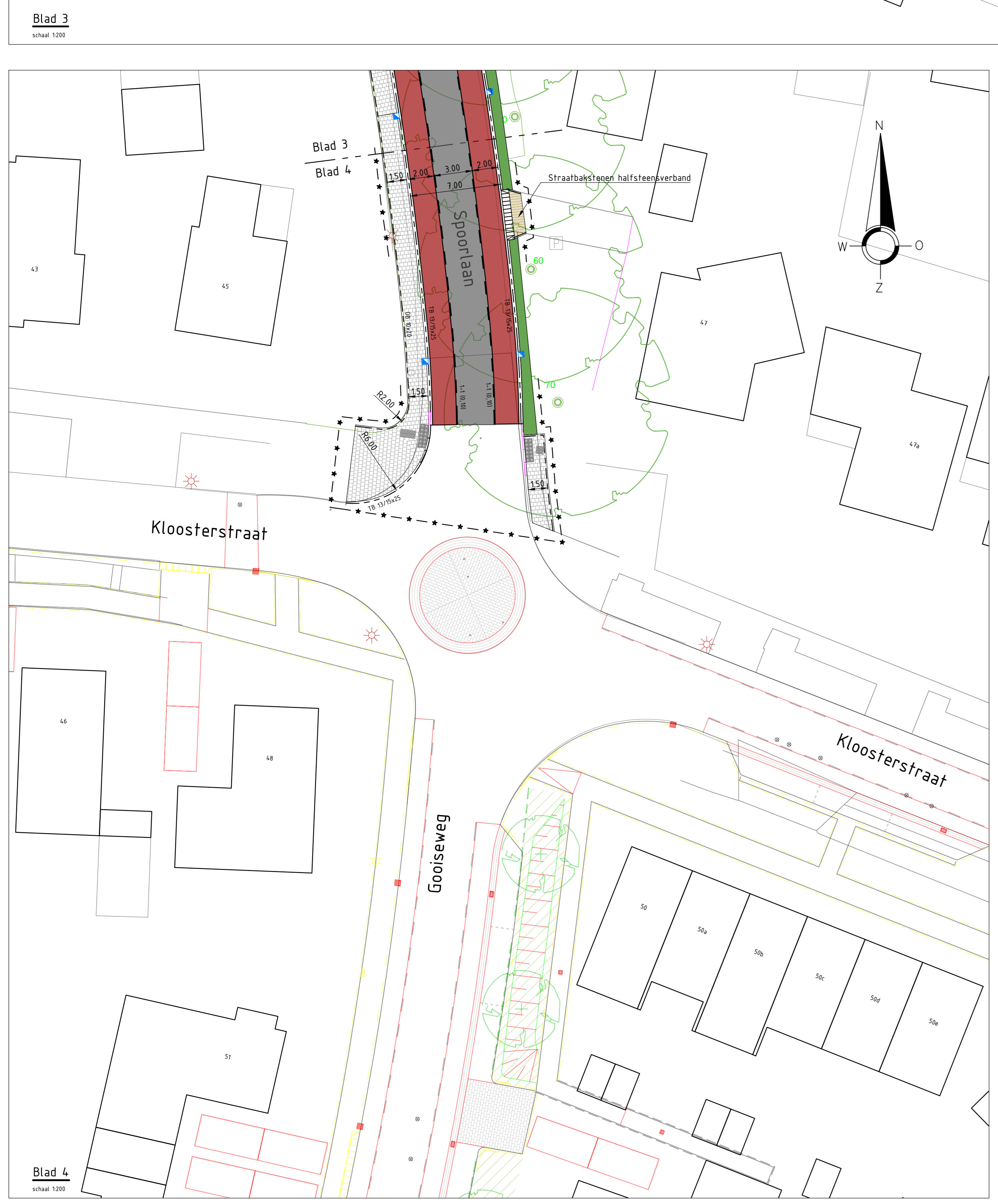
Blad 4 schaal 1:200
