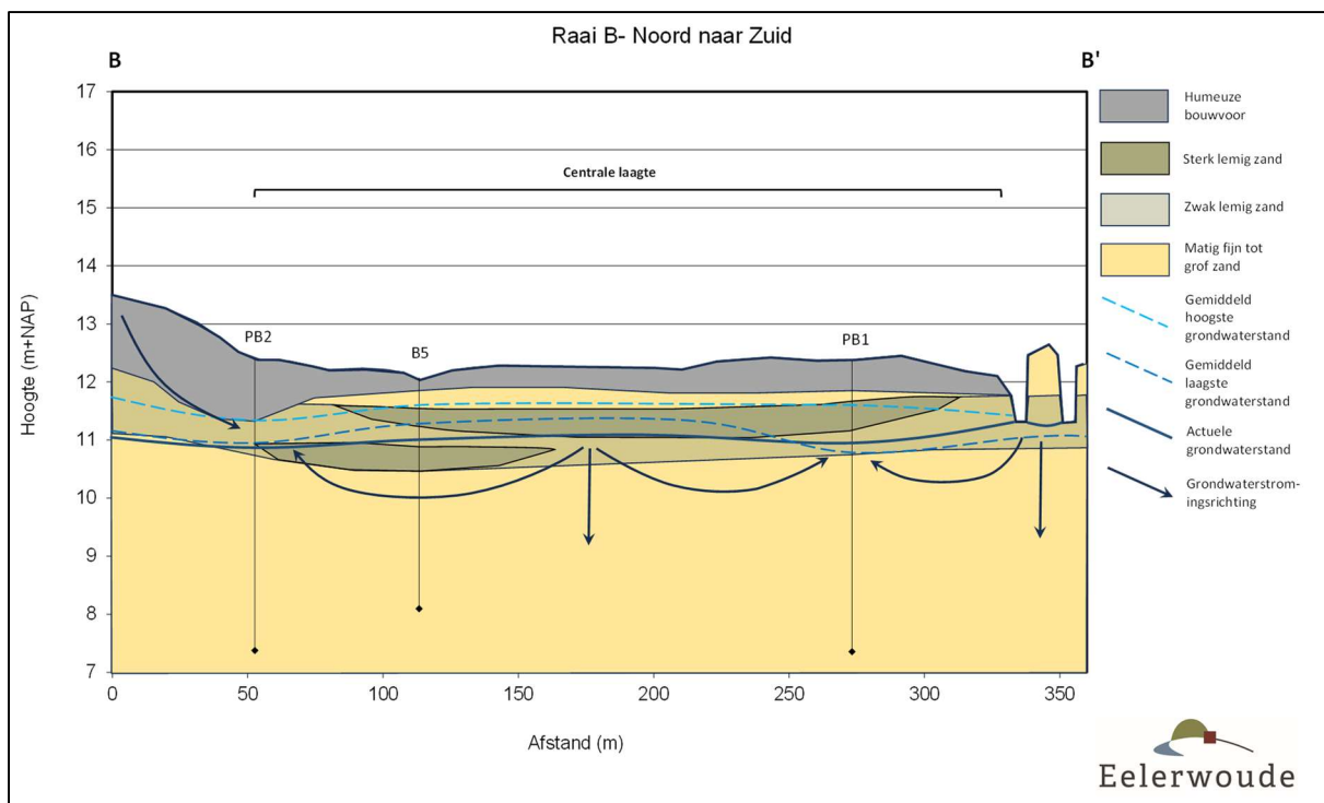
Figuur 6: lokale dwarsdoorsnede noord naar zuid
