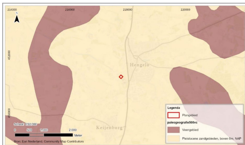
Afbeelding 3.1: Paleogeografische kaart 500 v.Chr. 4
