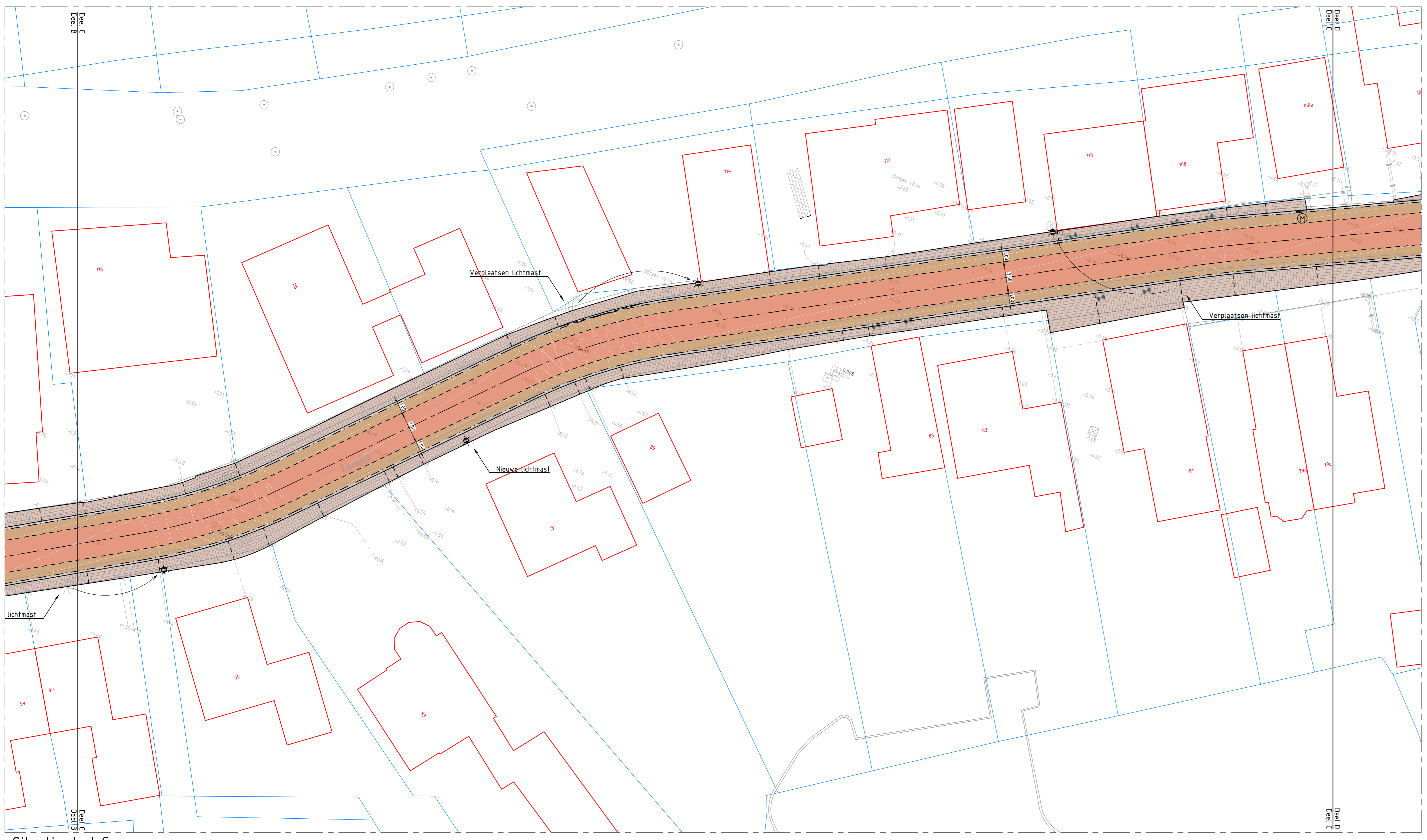
Situatie deel C schaal 1:200
