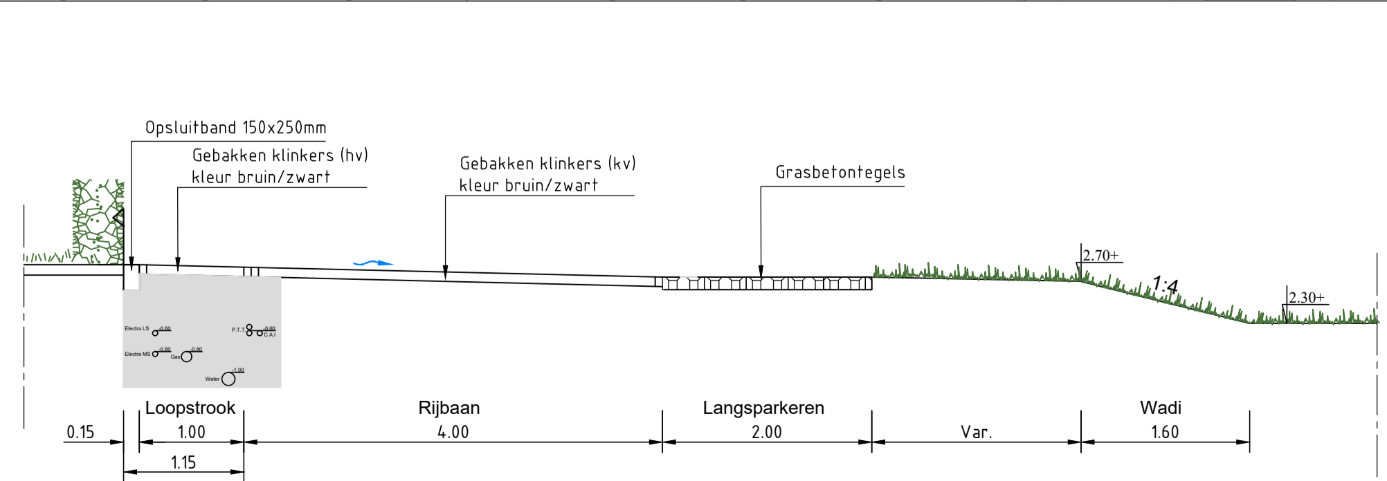
(Principe) dwarsprofiel 01 Schaal 1:50
