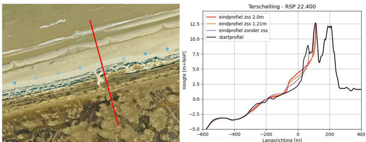
Figuur 17 Afslagprofielen voor Jarkusraai bij RSP 22.40 op het eiland Terschelling. Links is de locatie weergegeven in rood op een satellietbeeld uit 2023. Rechts het startprofiel in zwart en een afslagprofiel voor het huidige zichtjaar zonder zeespiegelstijging (paars), een afslagprofiel met 1,21m zeespiegelstijging in 2100 (oranje) en een afslagprofiel met 2,0m zeespiegelstijging in 2100 (rood). Met de iconen zijn de objecten aangegeven.
