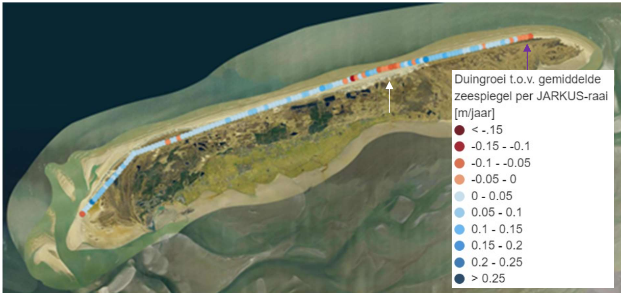
Figuur 22 Blokkendoos Levendige Kust – Duingroei t.o.v. 2 meter zeespiegelstijging per Jarkus-raai. Duingroei per raai is gedefinieerd (per strekkende meter) als een gemiddelde groei boven de 3m +NAP.
