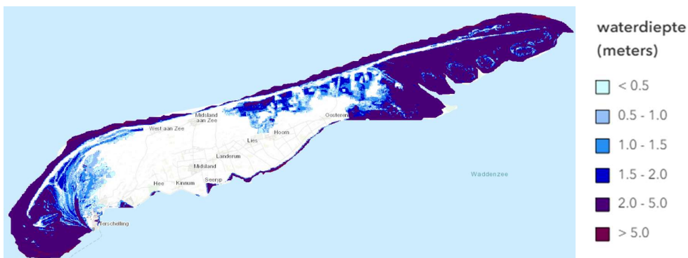
Figuur 27 Waterdiepte bij een 1/10.000 per jaar situatie in de huidige situatie. In 2100 komt deze situatie ongeveer 1/1.000pj voor. (NB: het overstroomde gebied is weergegeven op basis van de huidige normsituatie, in de situatie van 2100 zal er een verschil met waterdieptes van maximaal 1 m waterdiepte bij komen afhankelijk van de maaiveldhoogte < 0,5 en 0,5-1,0 m)
