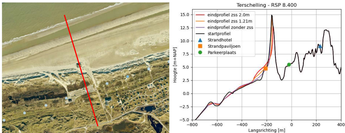
Figuur 16 Afslagprofielen voor Jarkusraai bij RSP 8.40 op het eiland Terschelling. Links is de locatie weergegeven in rood op een satellietbeeld uit 2023. Rechts het startprofiel in zwart en een afslagprofiel voor het huidige zichtjaar zonder zeespiegelstijging (paars), een afslagprofiel met 1,21m zeespiegelstijging in 2100 (oranje) en een afslagprofiel met 2,0m zeespiegelstijging in 2100 (rood). Met de iconen zijn de objecten aangegeven.
