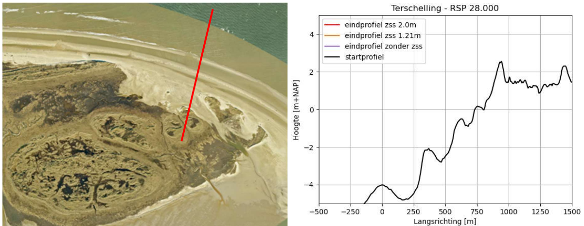
Figuur 18 Afslagprofielen voor Jarkusraai bij RSP 28.00 op het eiland Terschelling. Links is de locatie weergegeven in rood op een satellietbeeld uit 2023. Rechts het startprofiel in zwart en een afslagprofiel voor het huidige zichtjaar zonder zeespiegelstijging (paars), een afslagprofiel met 1,21m zeespiegelstijging in 2100 (oranje) en een afslagprofiel met 2,0m zeespiegelstijging in 2100 (rood). Met de iconen zijn de objecten aangegeven.
