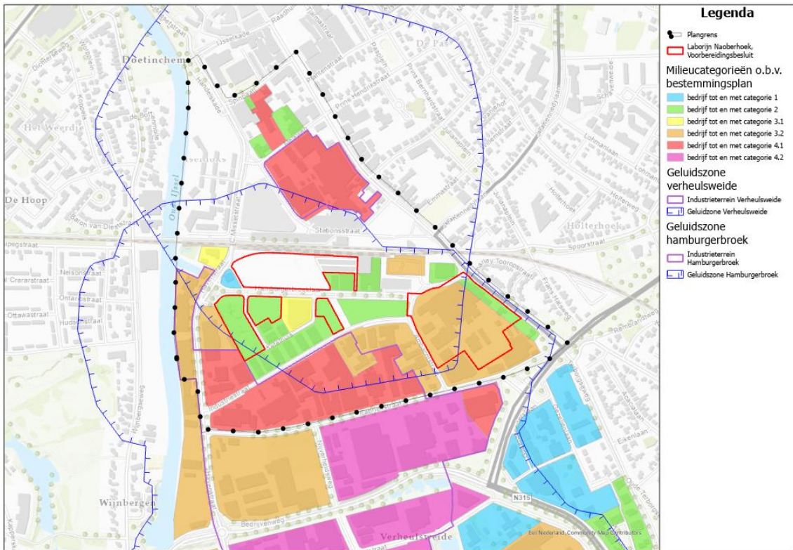
Geluidszones bedrijventerreinen
