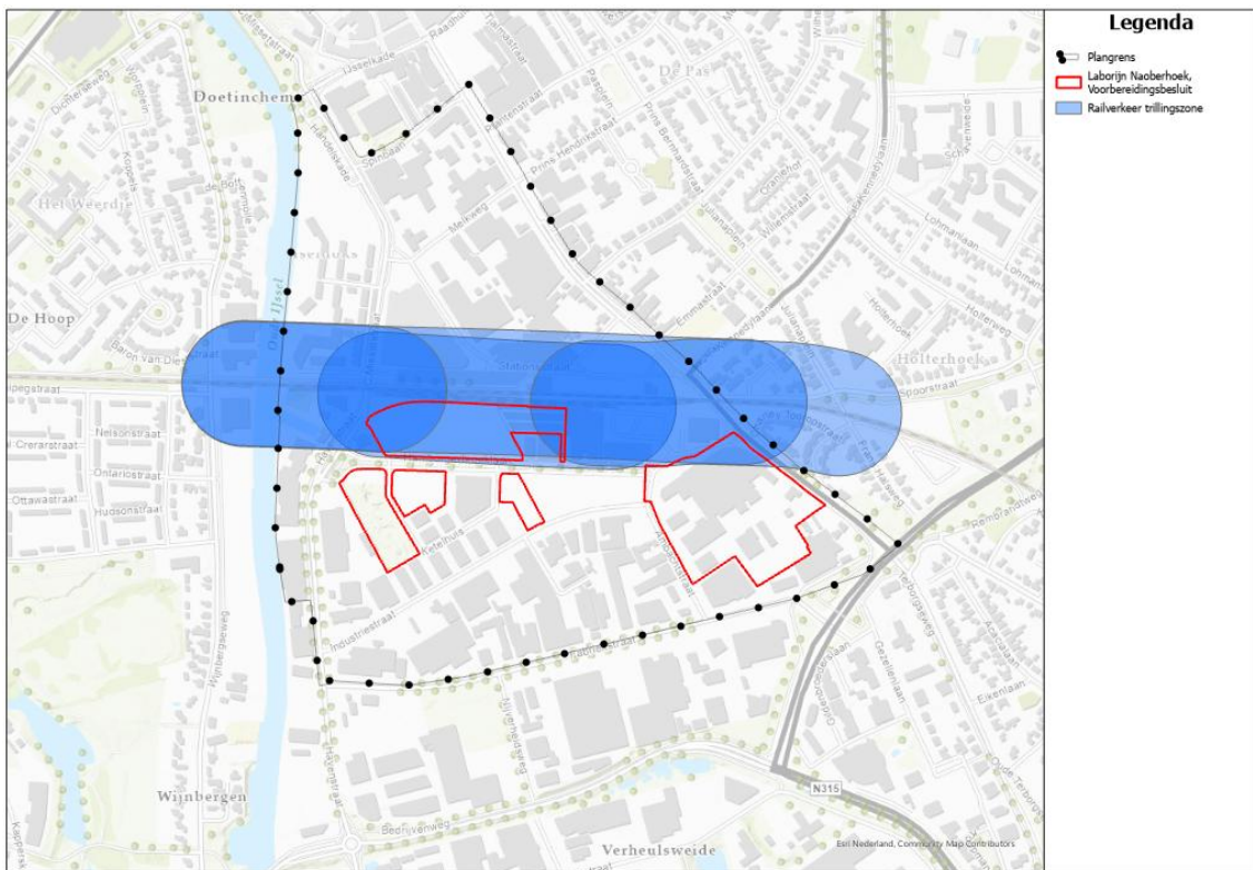
Trillingszone spoorwegen
