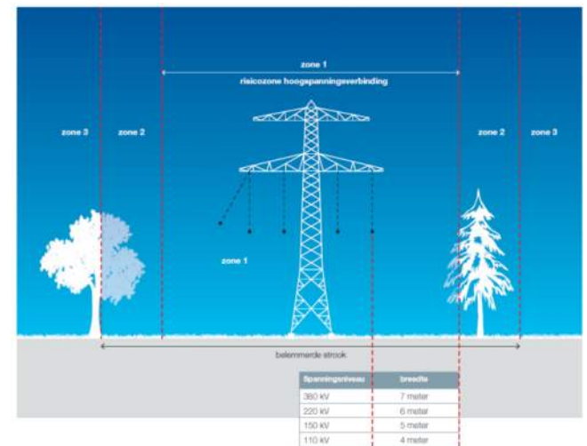
Schema risicozones rond hoogspanningsverbindingen. Bron: Document Tennet – "Gedragscode houtopstanden en hakhoutbeheer"
