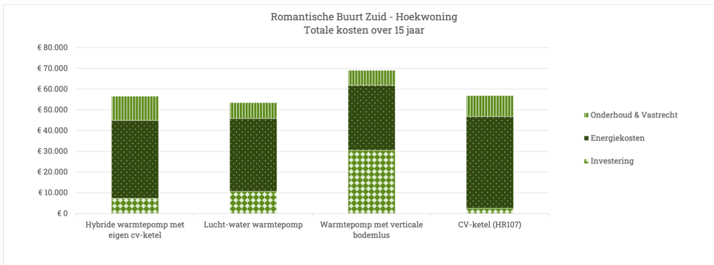
Figuur 12a en 12b Totale kosten voorbeeldwoningen over 15 jaar voor een woningtype voor elke buurt, in vergelijking met de situatie met aardgas (rechter balk). De brochure waar deze grafieken in staan is in Bijlage 2 opgenomen
