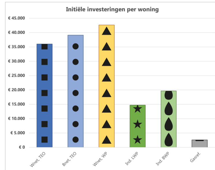
Figuur 4 Initiële investering per woning
