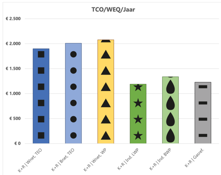
Figuur 3 Total cost of ownership (totale kosten voor de eigenaar en gebruiker). Legenda in tabel na volgende afbeelding
