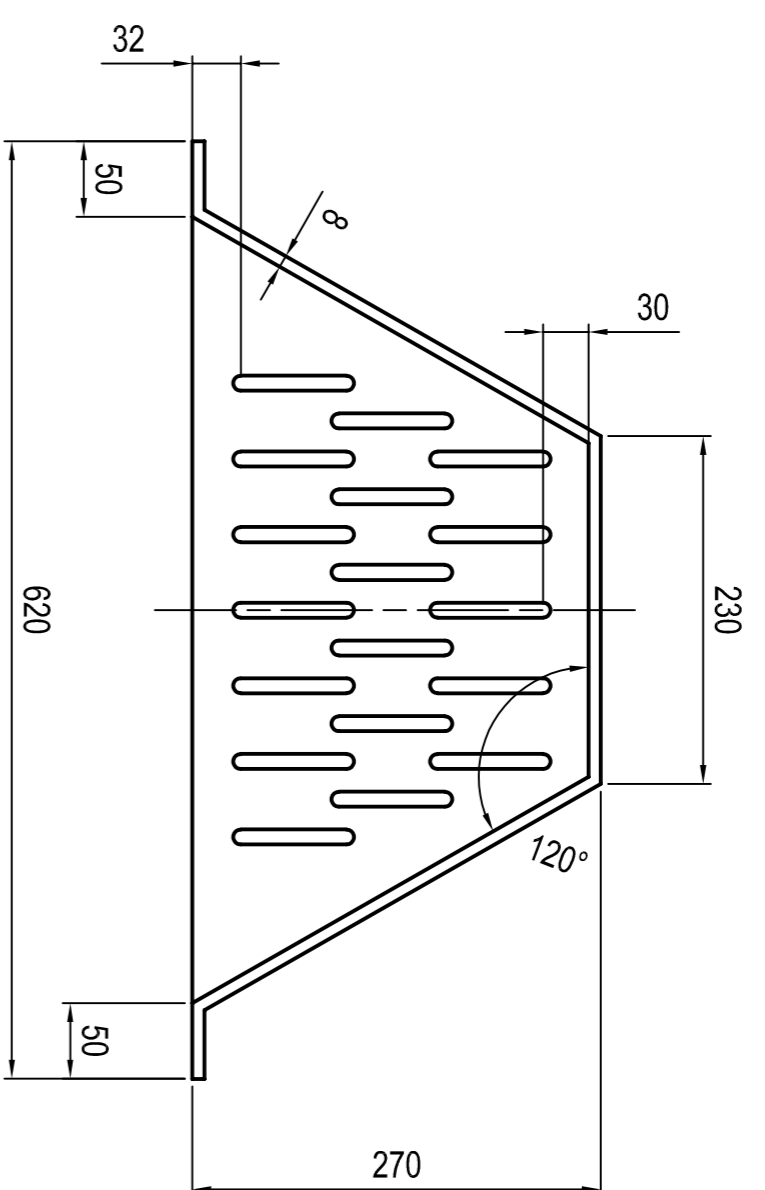
BOVENAANZICHT (zonder dekse)
