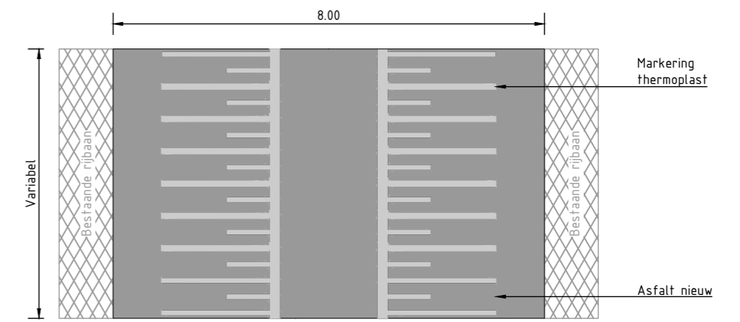
Principedetail 002: Verkeersdrempel 60km/uur H=8cm schaal 1:100
