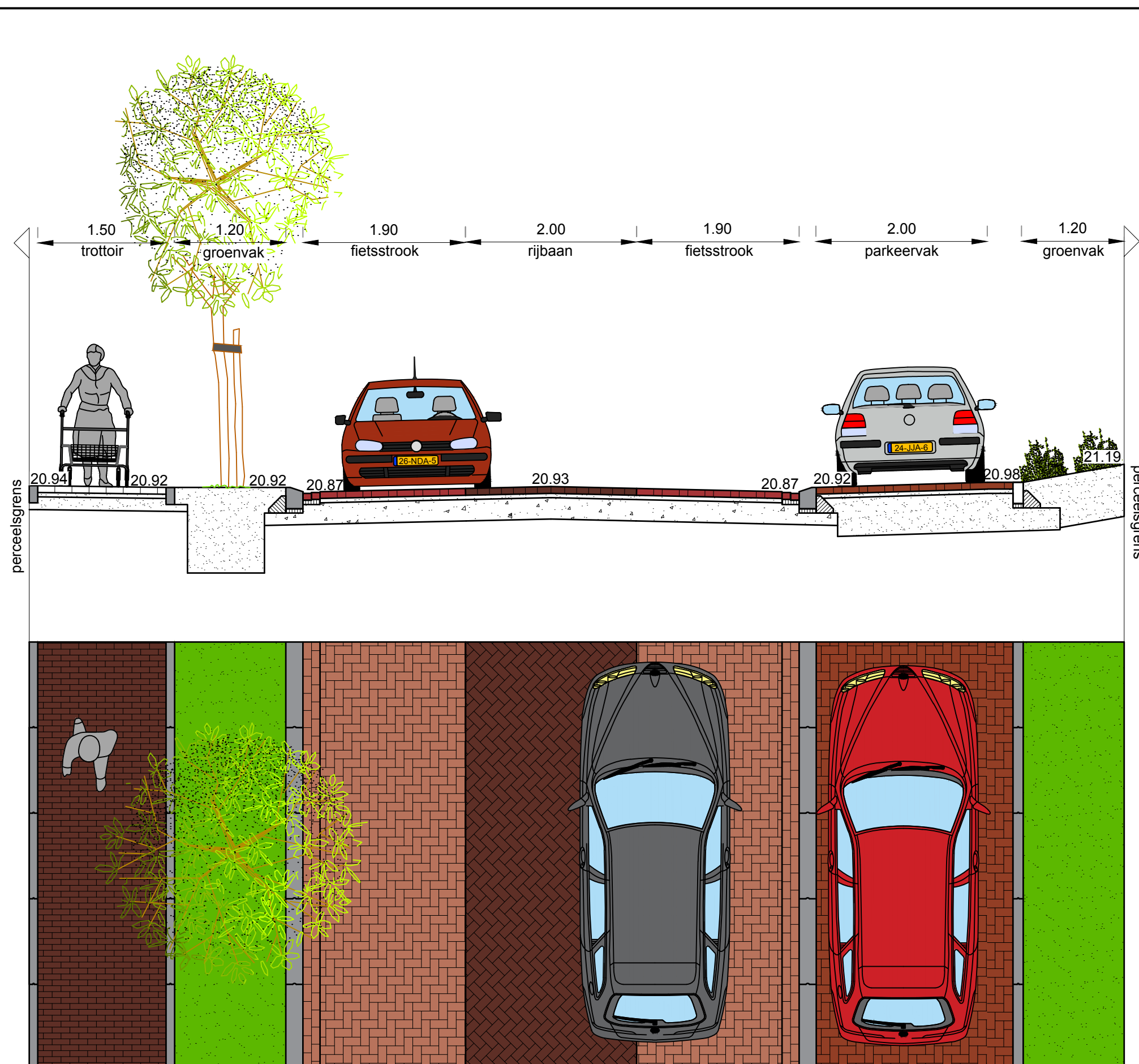
Dwarsprofiel D-D schaal: 1 : 50
