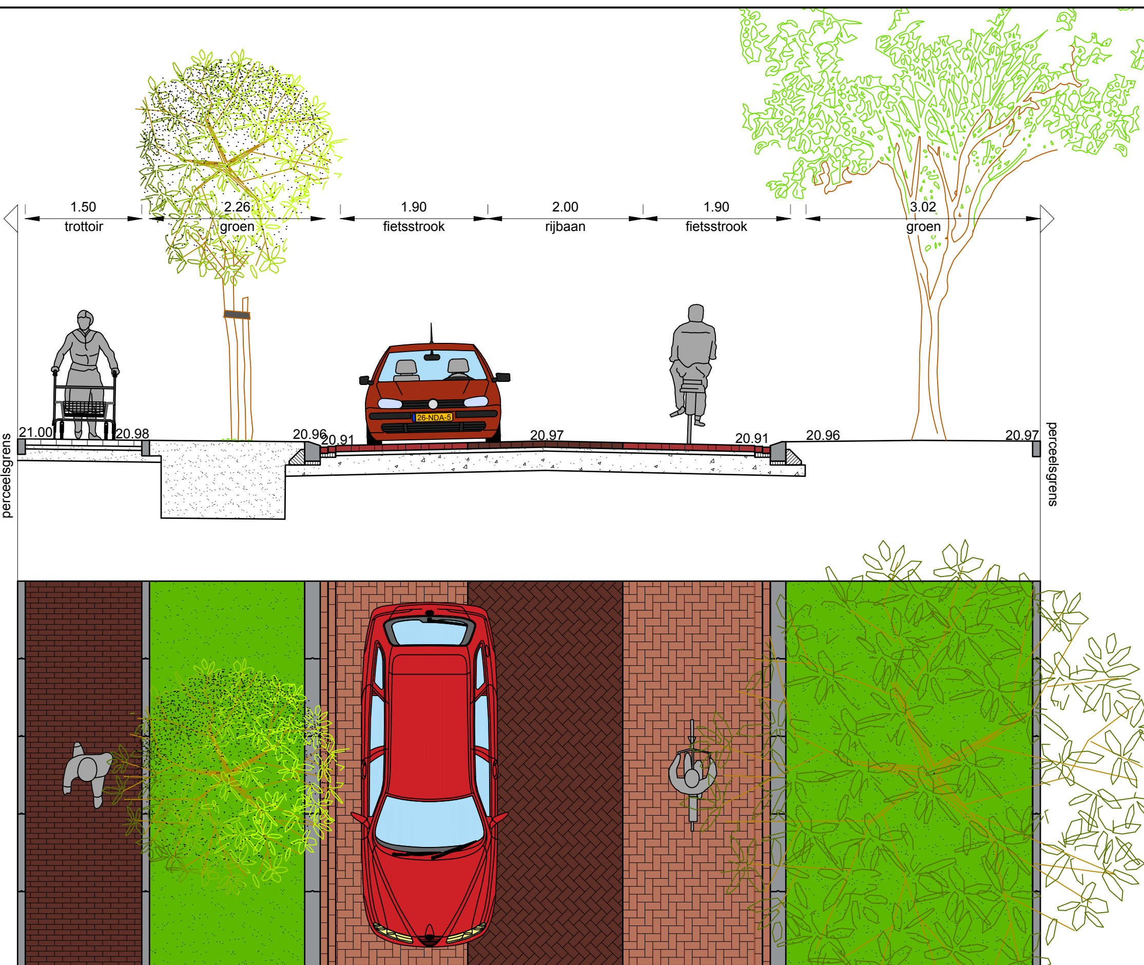
Dwarsprofiel C-C schaal: 1 : 50
