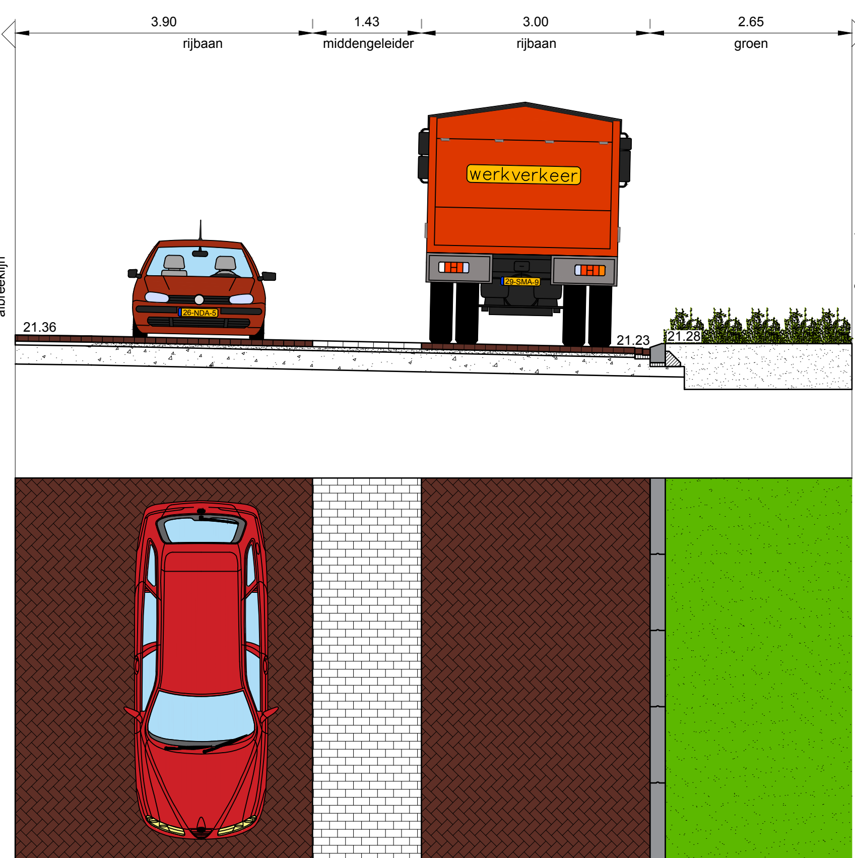
Dwarsprofiel A-A schaal: 1 : 50
