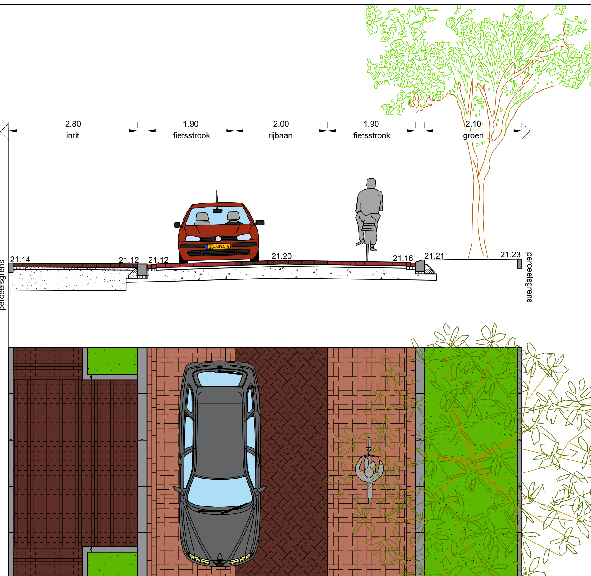
Dwarsprofiel B-B schaal: 1 : 50
