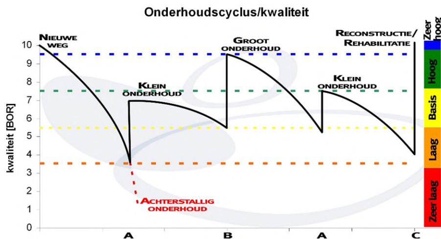
Figuur 5-1: Schematische voorstelling van verloop in wegkwaliteit
