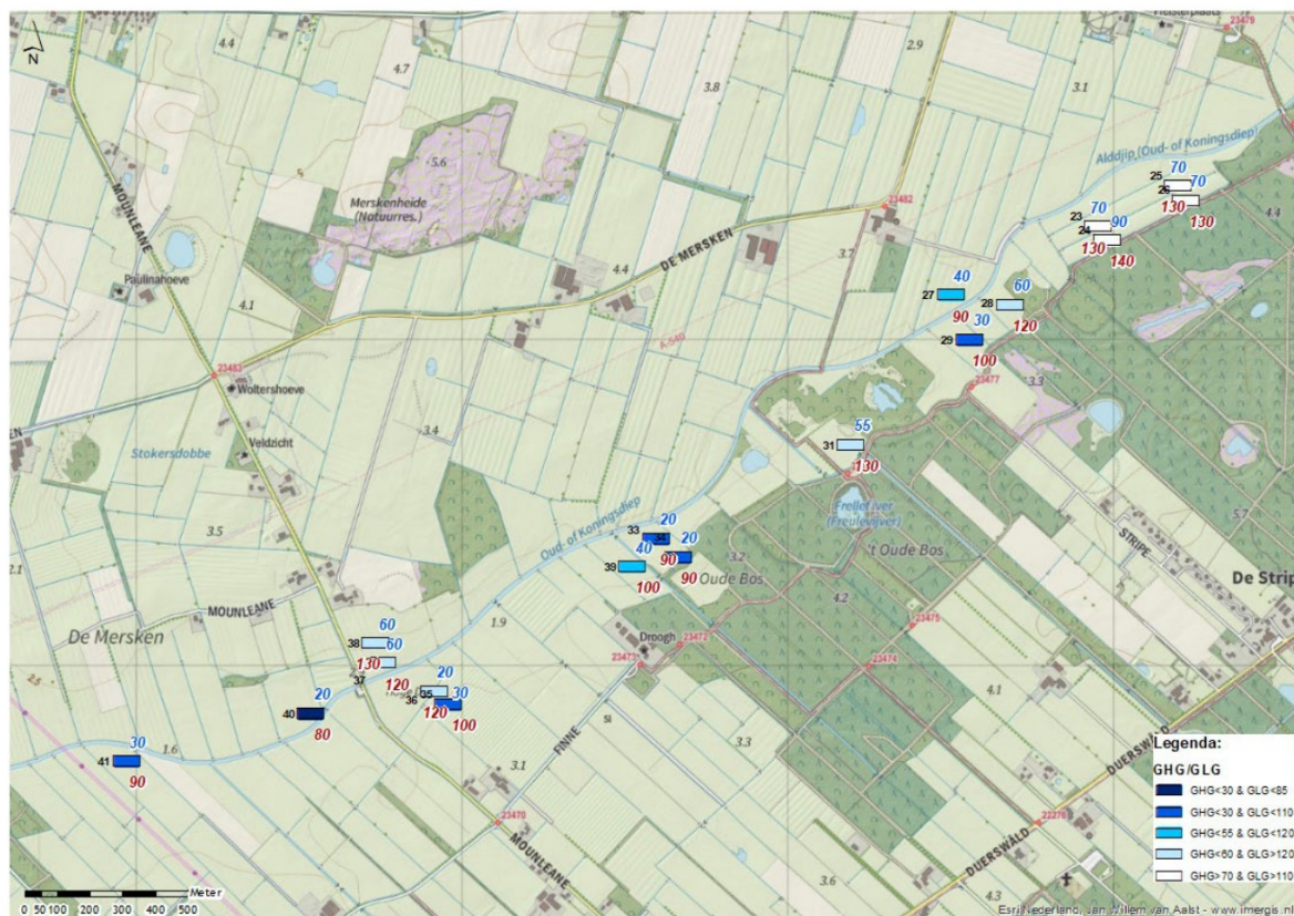
Figuur 19. Overzicht van de afgeleide grondwaterstanden (GHG boven in blauw en GLG onder in rood) per locatie in de deelgebieden Mounleane Oost en West. Alleen de locaties bemonsterd door ATKb zijn opgenomen omdat hier de grondwaterstanden zijn afgeleid aan de hand van het boorprofiel.
