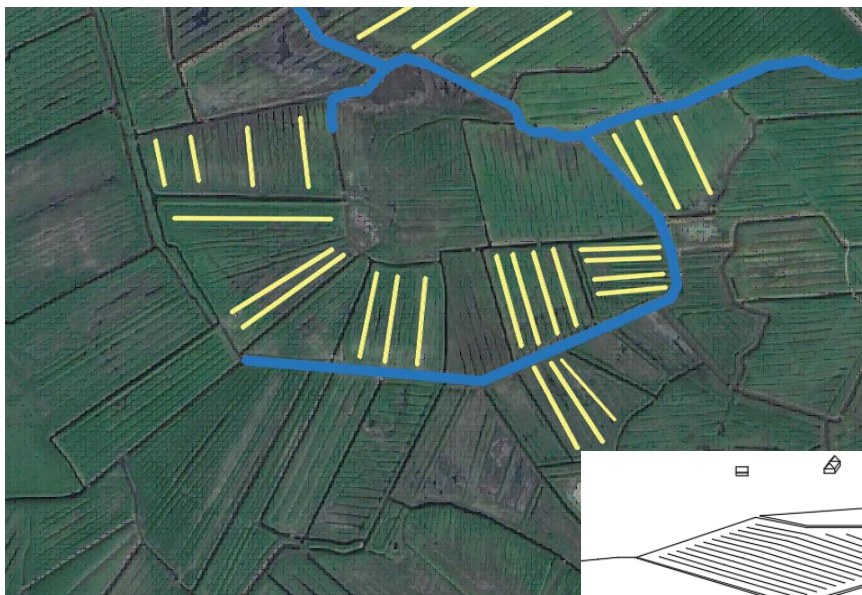
Richting van de greppels t.o.v. de hoofdwatgangen in een gebied
