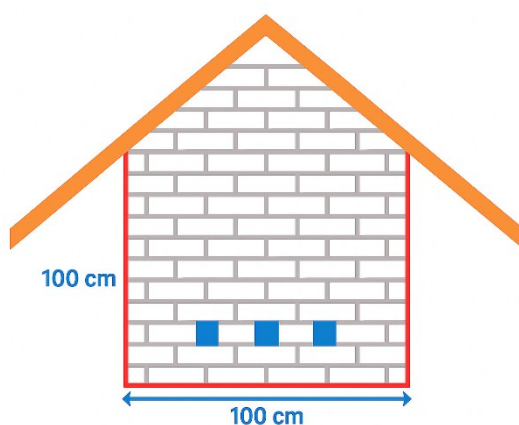
Figuur 7 Vooraanzicht spouwverblijf in kopgevel met locaties invliegopeningen (blauw). Hetzelfde principe geldt voor een klein spouwverblijf bij een tussenwoning, met de aangepaste afmetingen 30 x 30 cm.
