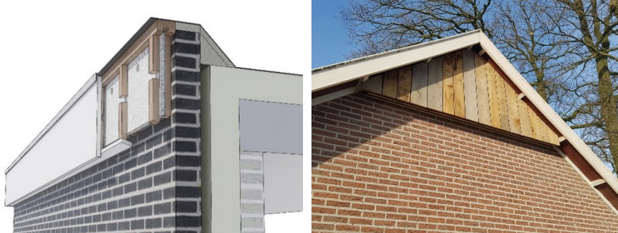
Figuur 12 Voorbeeld van natuurinclusieve oplossingen voor vleermuizen: links verblijfplaatsen in/onder dakrand, rechts: betimmering bij nok.
