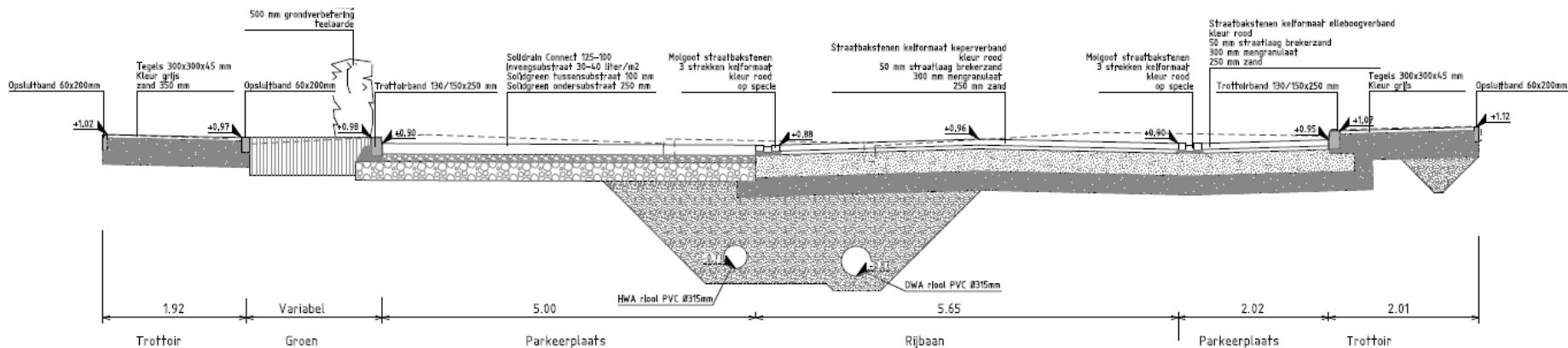
Doorsnede C-C
