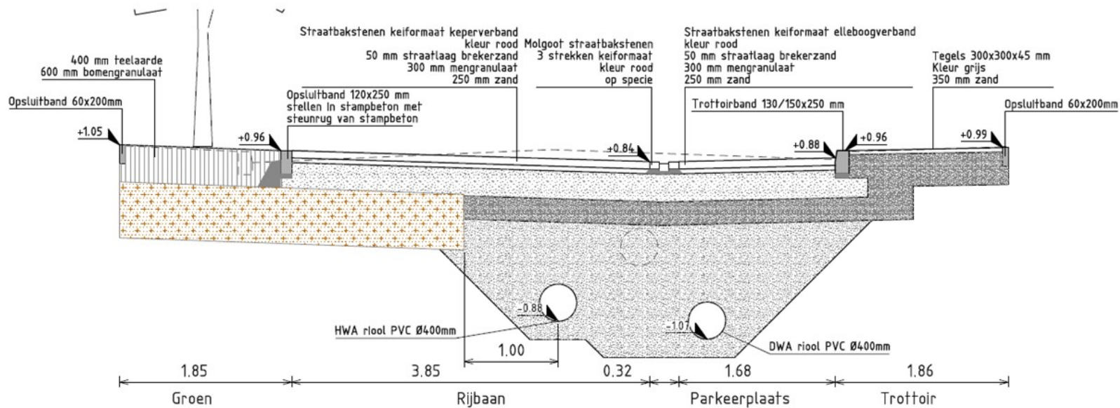
Doorsnede B-B
