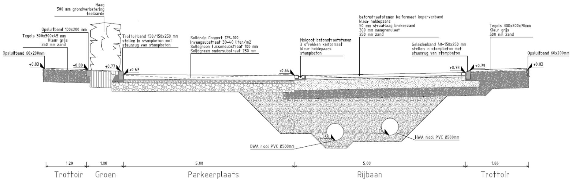
Doorsnede A-A
