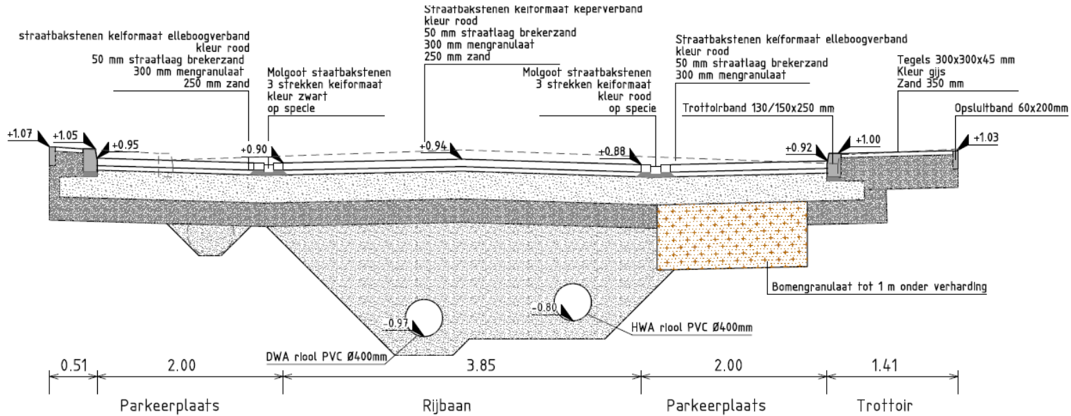
Doorsnede D-D
