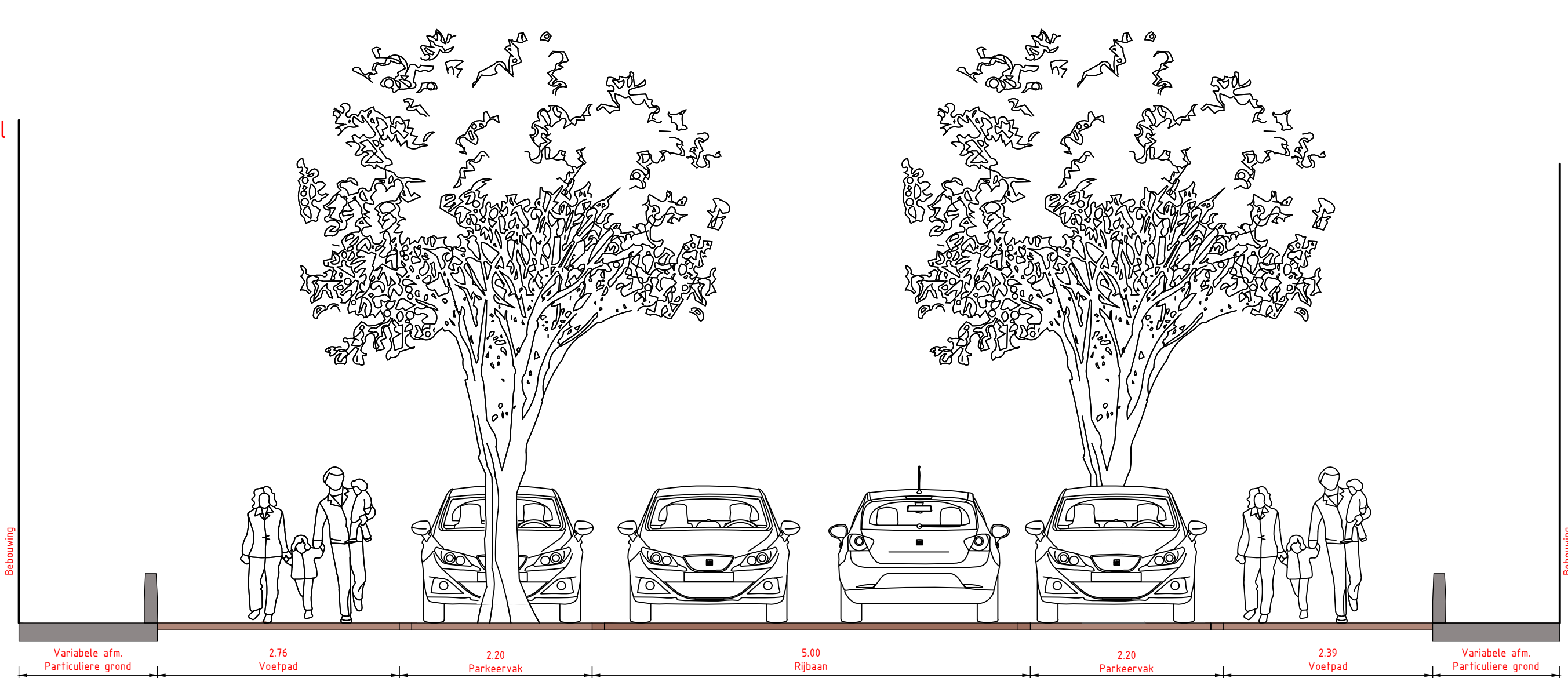
Principe Profiel 1:50 A-A
