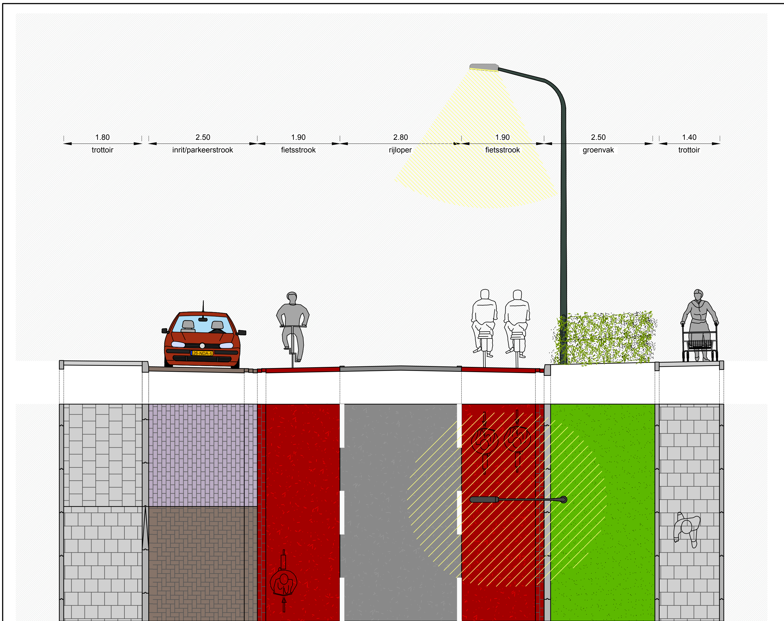
Dwarsprofiel A-A schaal: 1 : 50
