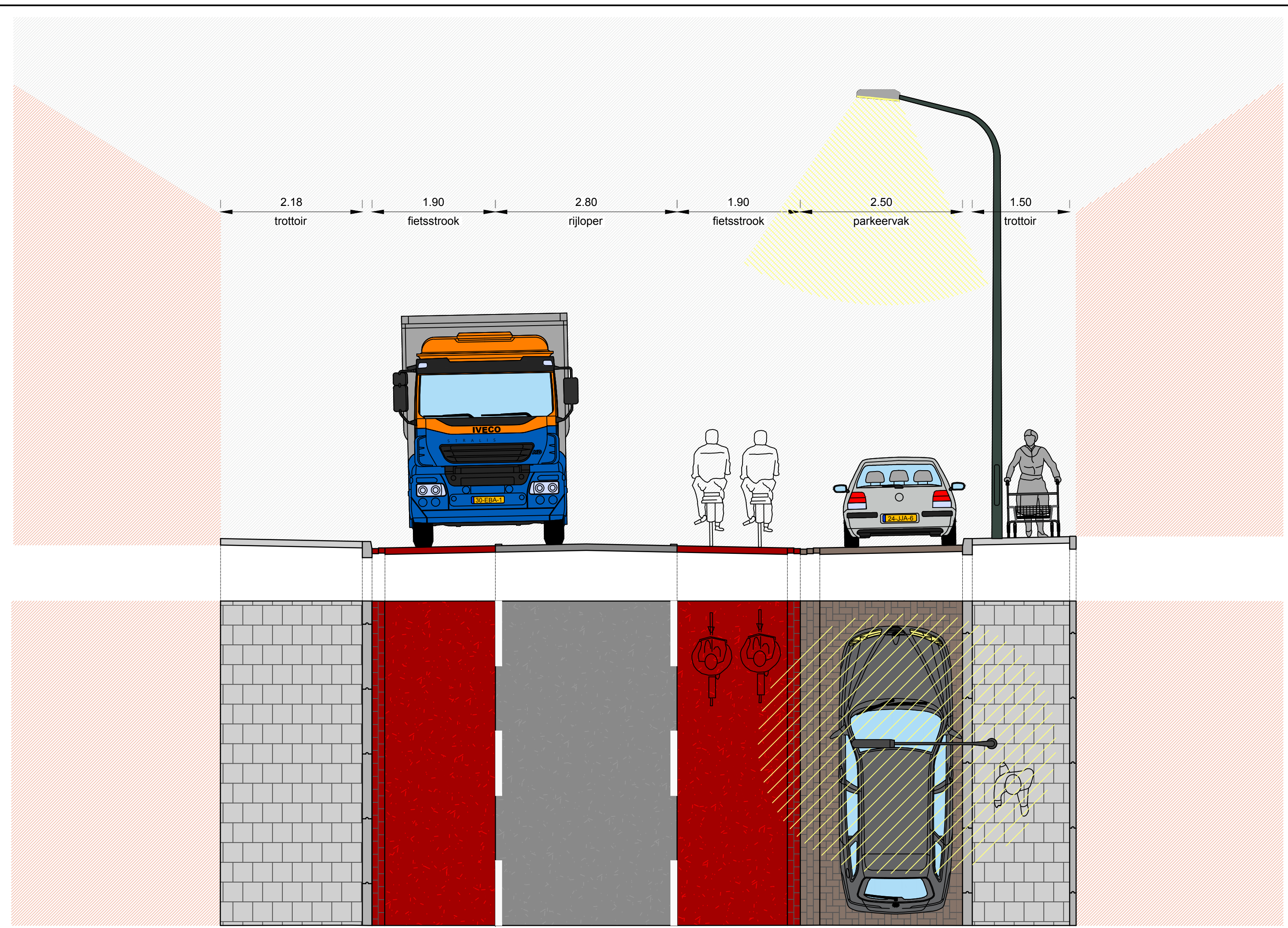
Dwarsprofiel B-B schaal: 1 : 50
