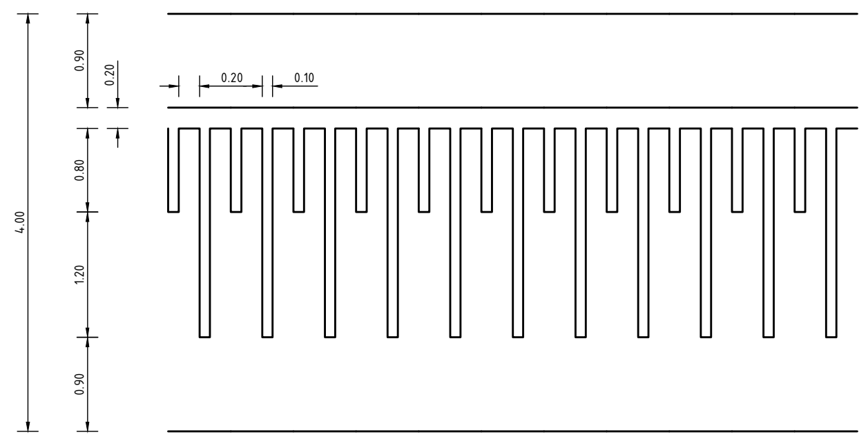
Aanzicht sinus drempel Schaal 1 : 50
