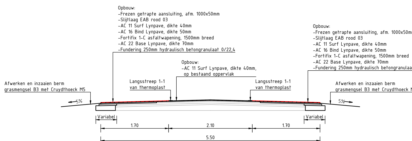
Profiel nieuwe situatie Schaal 1 : 50
