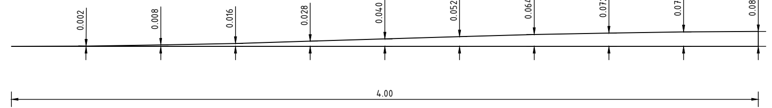
Dwarsprofiel sinus drempel Schaal 1 : 20
