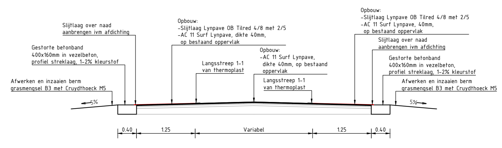
Profiel nieuwe situatie Schaal 1:50
