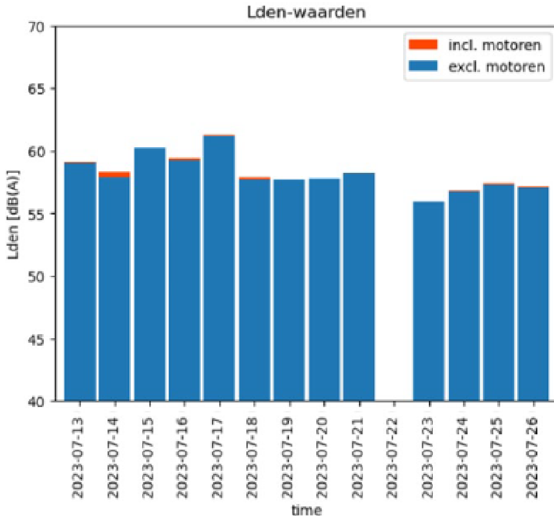
Figuur 3-2: Daggemiddelden inclusief en exclusief motoren
