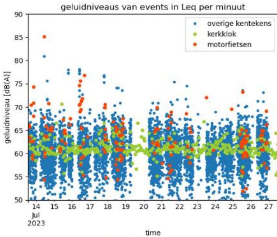
Figuur 3-1: Geluidsniveau van verschillende 'gebeurtenissen'
