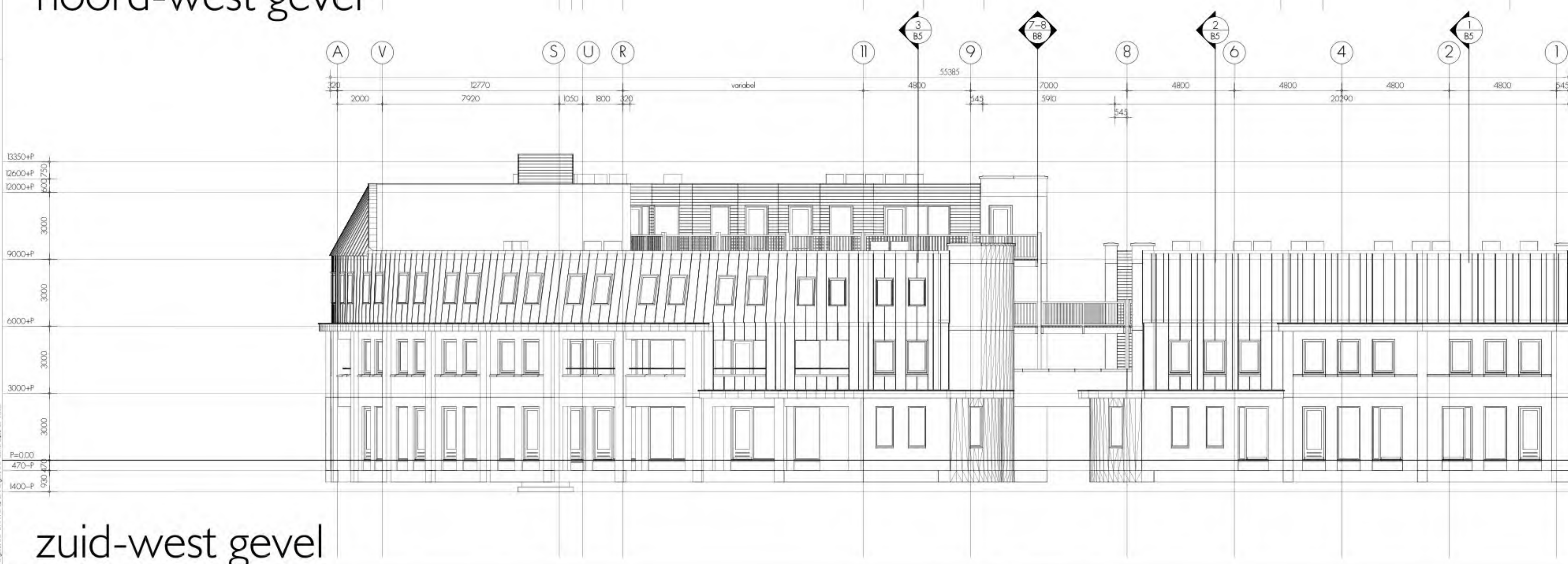
noord-west gevel
