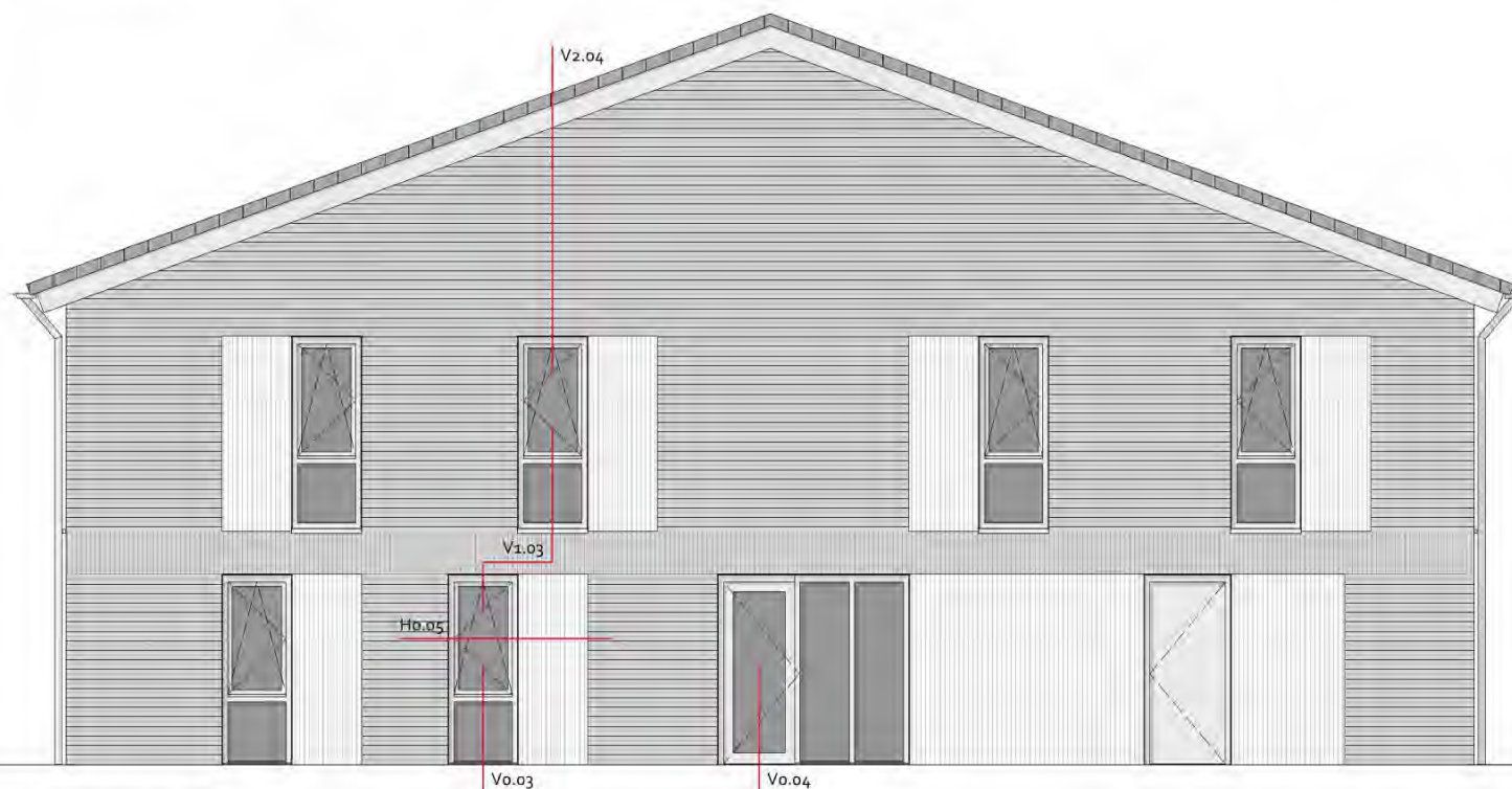
voorgevel
