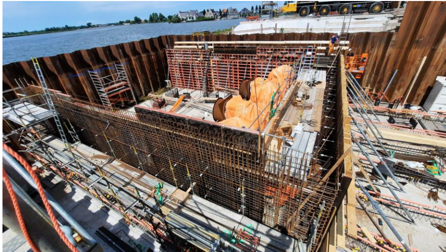
Foto 4: jul '22 wapening wanden instroomzijde
