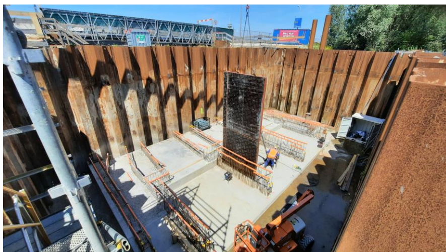
Foto 3: jun '22 vloer uitstroomzijde
