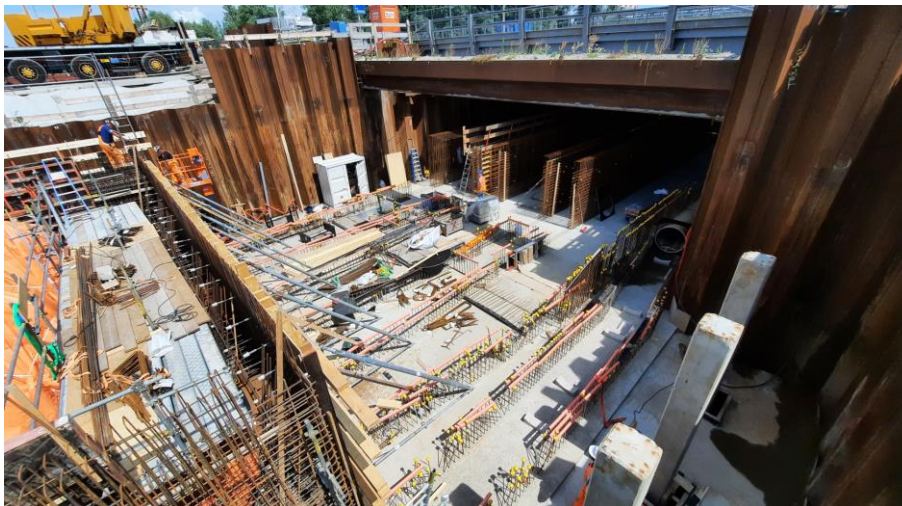
Foto 5: jul '22 wapening wanden weggedeelte
