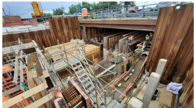
Foto 11 en 12: sep '22 houten trompetstukken worden ingehesen en geplaatst
