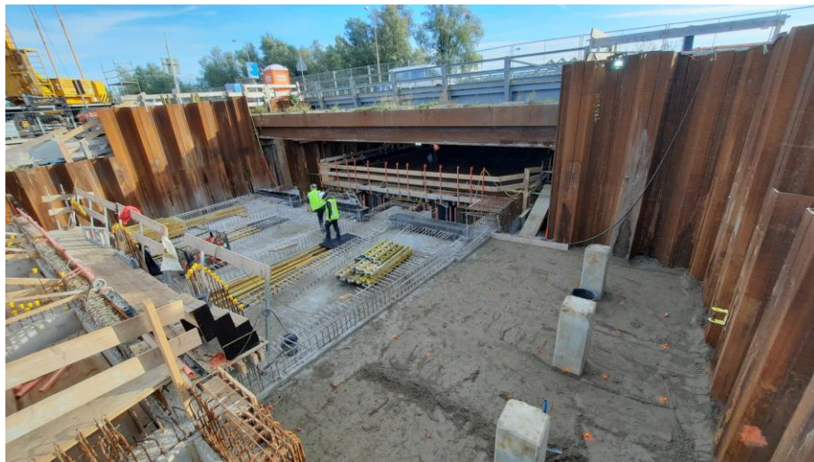
Foto 18: eind okt '22 trompetstukken tussen pomp en maalgang zijn omhuld met beton en ook is gestart met grondwerk bovenop restant vispassage.
