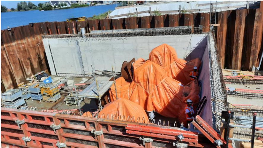
Foto 7: aug '22 gestorte wanden instroom
