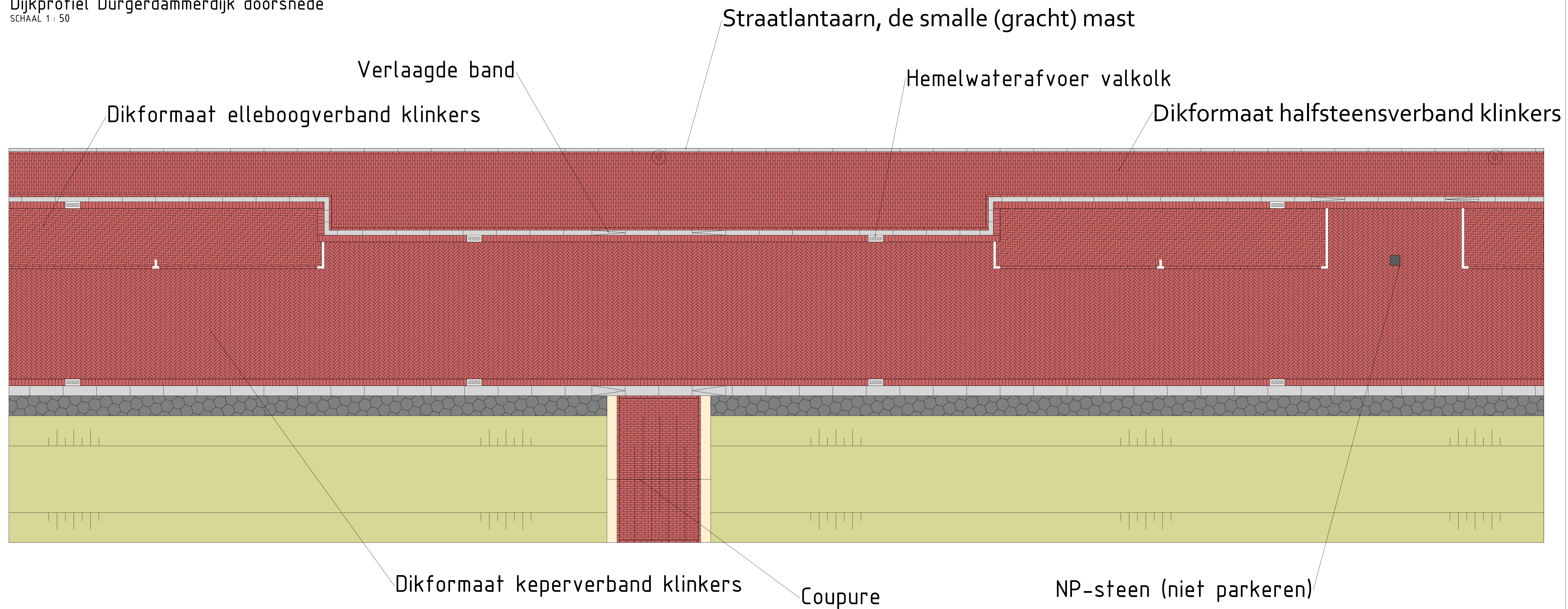
Dijkprofiel Durgerdammerdijk detail uitwerking SCHAAL 1 : 50
