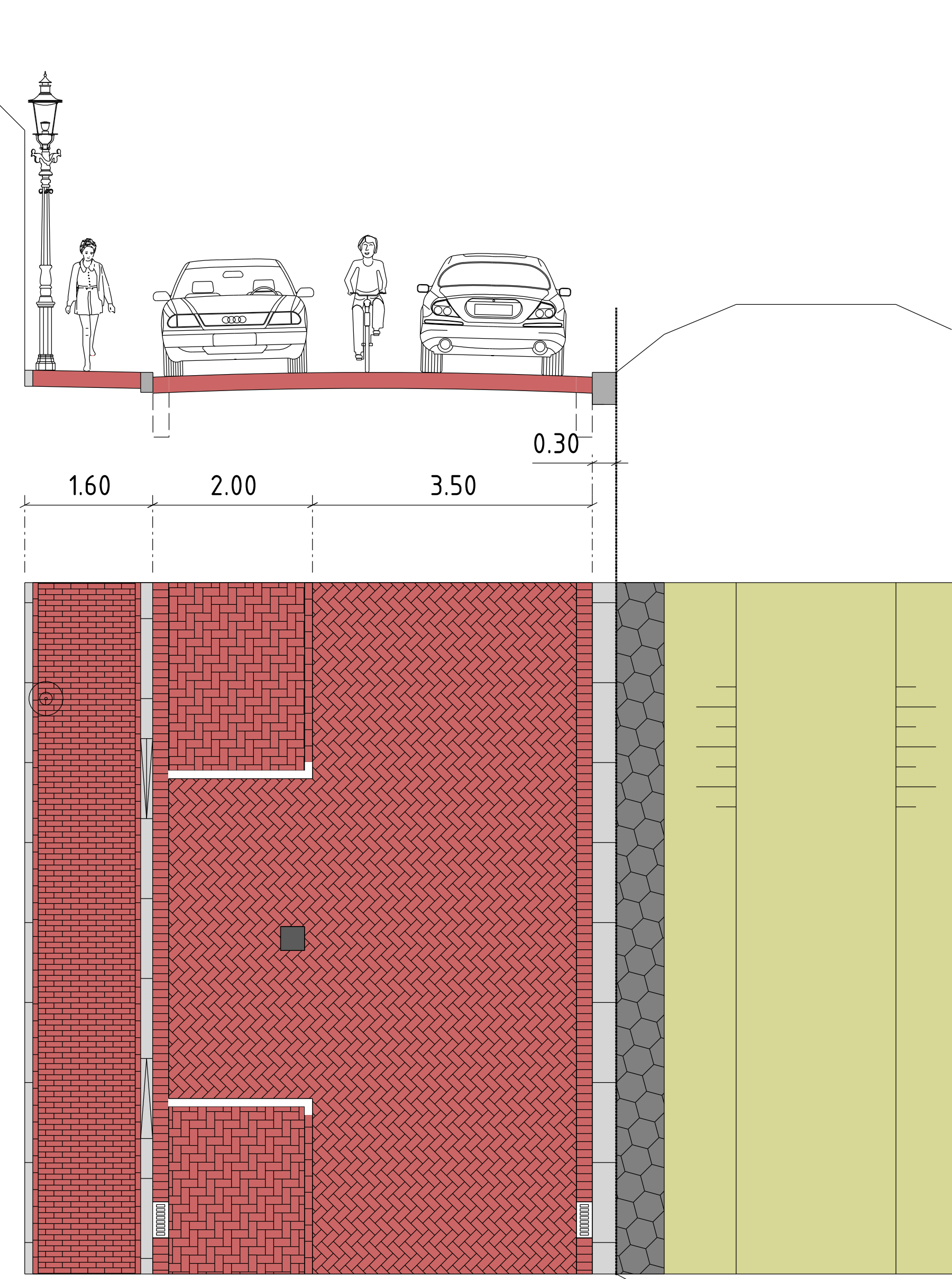
Dijkprofiel Durgerdammerdijk doorsnede SCHAAL 1 : 50
