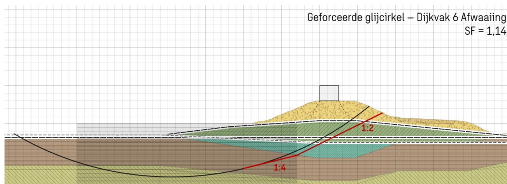
Figuur 4-6 Afschuiving (zwarte lijn) en vervolgafschuiving (rode lijn) na forceren van grotere glijcirkel
