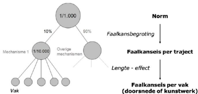
Figuur 2-4: Bepalen van de faalkanseis per toetsspoor en per vak [3]
