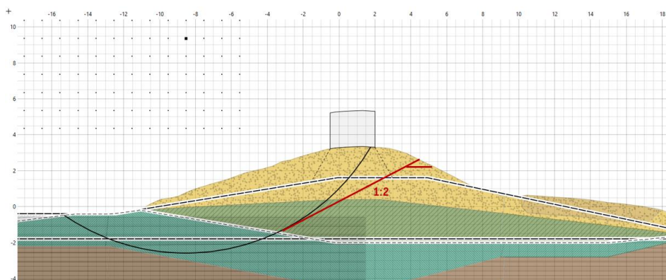
Figuur 4-5 Afschuiving (zwarte lijn) dijkvak 5 bij scenario regenval met vervolgafschuivingen (rode lijn)
