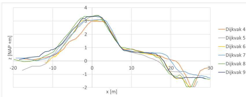
Figuur 3-9: Maatgevend dwarsprofiel per dijkvak, uitgelijnd op het knikpunt van binnentalud en berm
