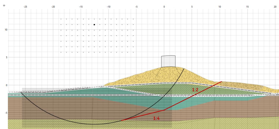
Figuur 4-3 Afschuiving (zwarte lijn) dijkvak 5 bij scenario afwaaiing met vervolgafschuivingen (rode lijn)
