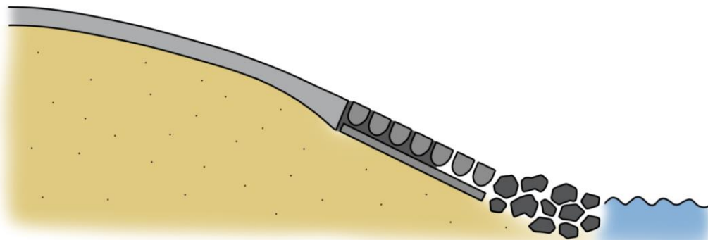
4. Steenzetting dichtgieten en teen open laten
