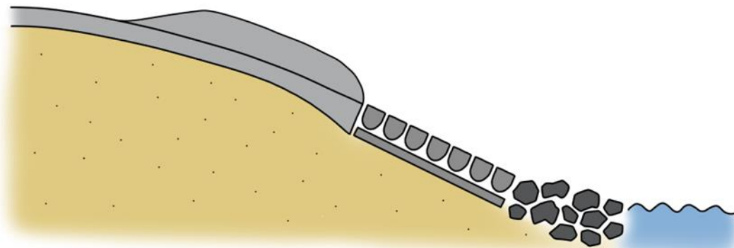
5. Asfaltbekleding overlagen met asfalt
