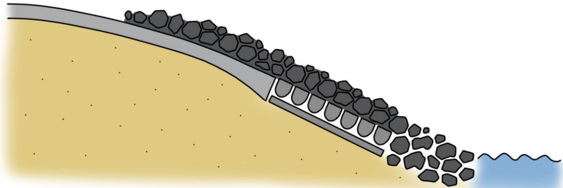
10. Asphalt- en zetsteenbekleding overlagen met gepenetreerde breuksteen
