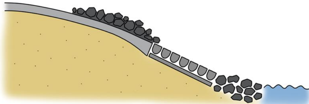
8. Asfaltbekleding overlagen met gepenetreerde breuksteen
