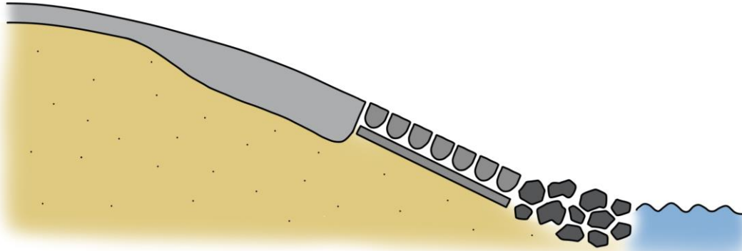
6. Asfaltbekleding vervangen door een dikkere asfaltbekleding
