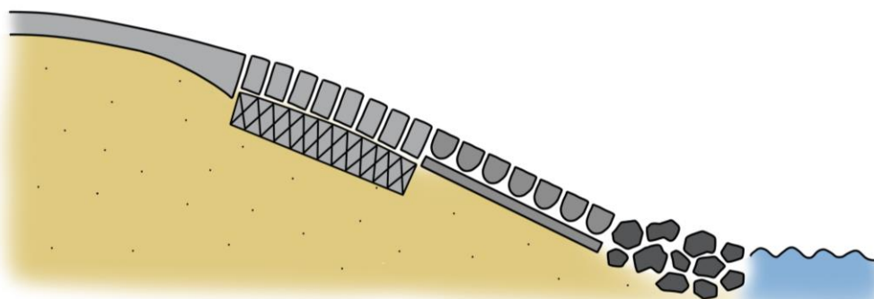
2. Asfaltbekleding vervangen door steenbekleding op ondoorlatende fundering
