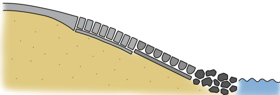
1. Asfaltbekleding vervangen door steenbekleding op open fundering
