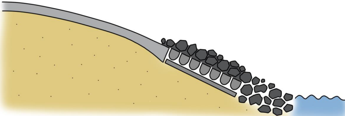
9. Steenzetting overlagen met gepenetreerde breuksteen
