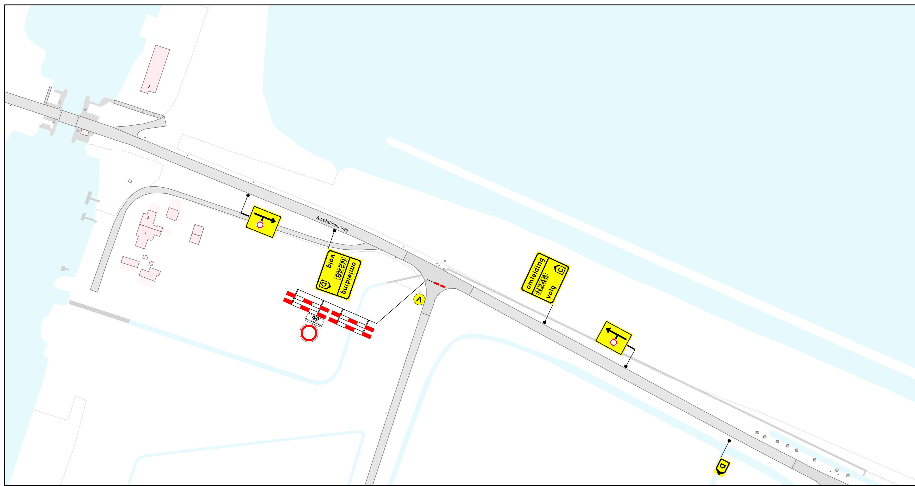
DETAIL 1 SCHAAL 1:1000
