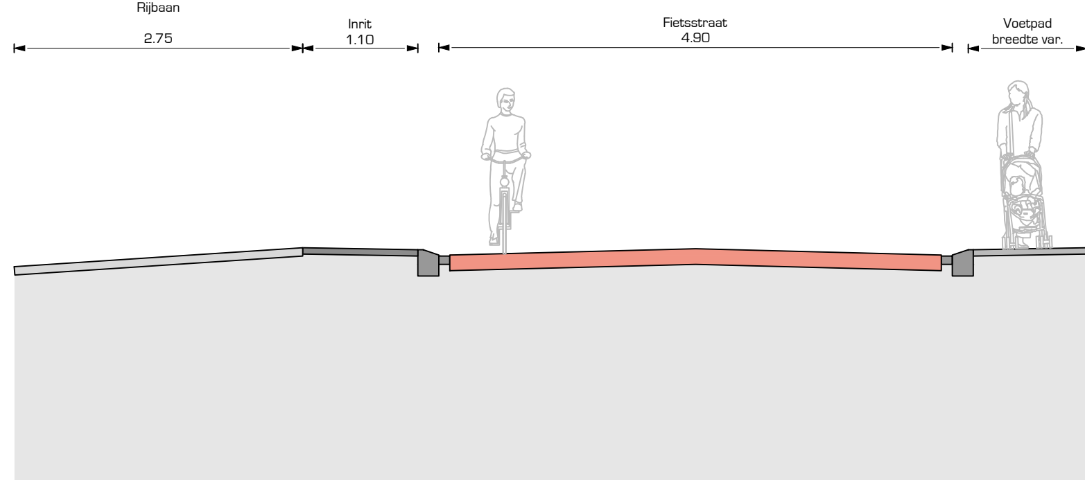
Dwarsprofiel C Schaal: 1:50
