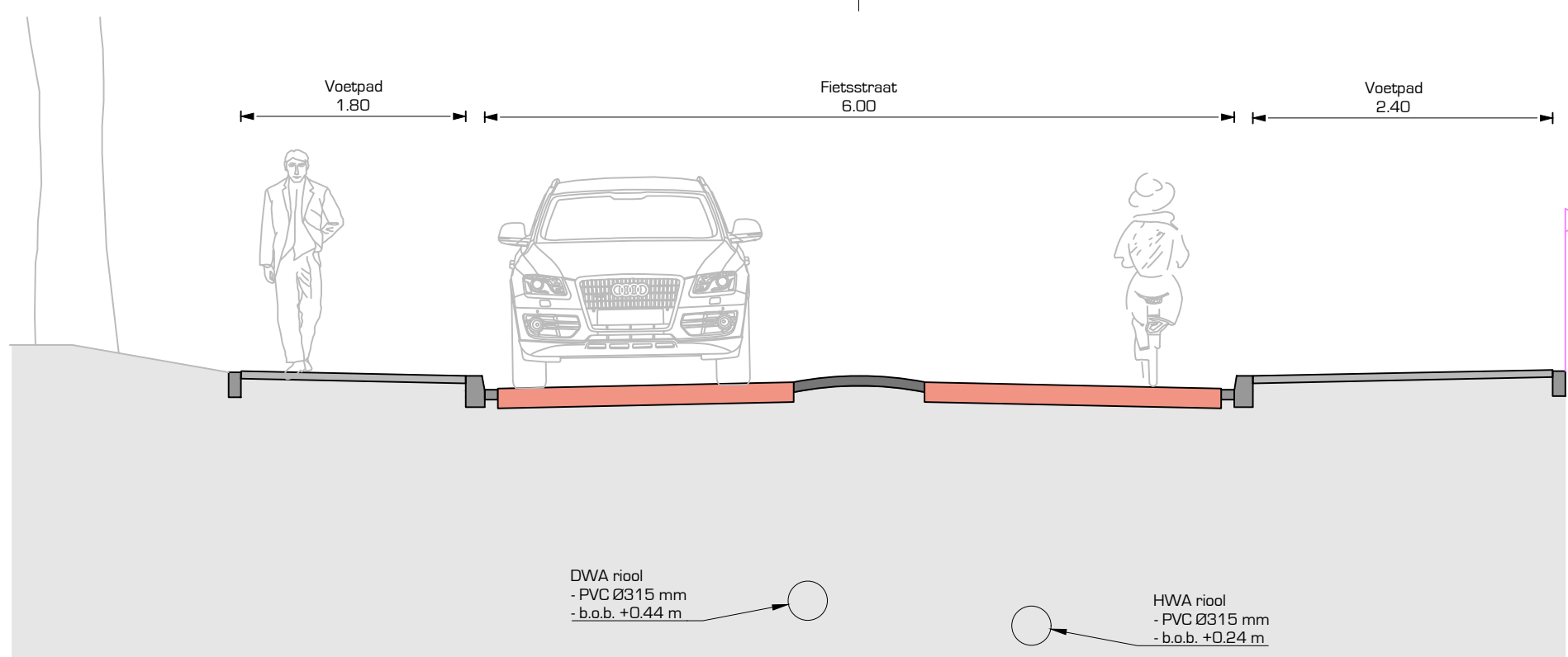
Dwarsprofiel A Schaal: 1:50
