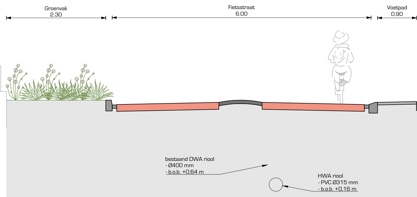
Dwarsprofiel B Schaal: 1:50
