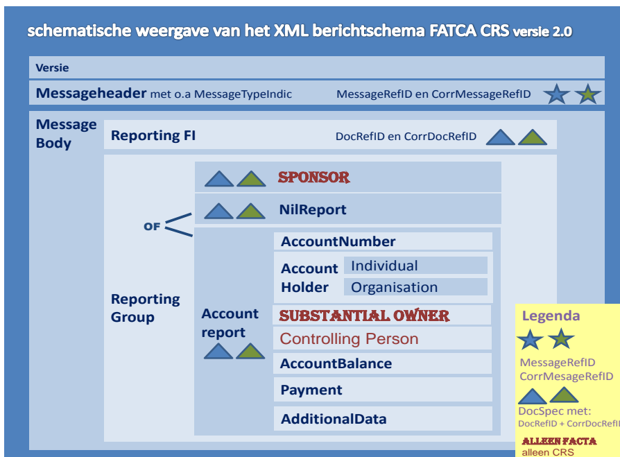
Figuur 3a; visualisatie van de structuur van het FATCA CRS XML berichtschema versie 2.0
