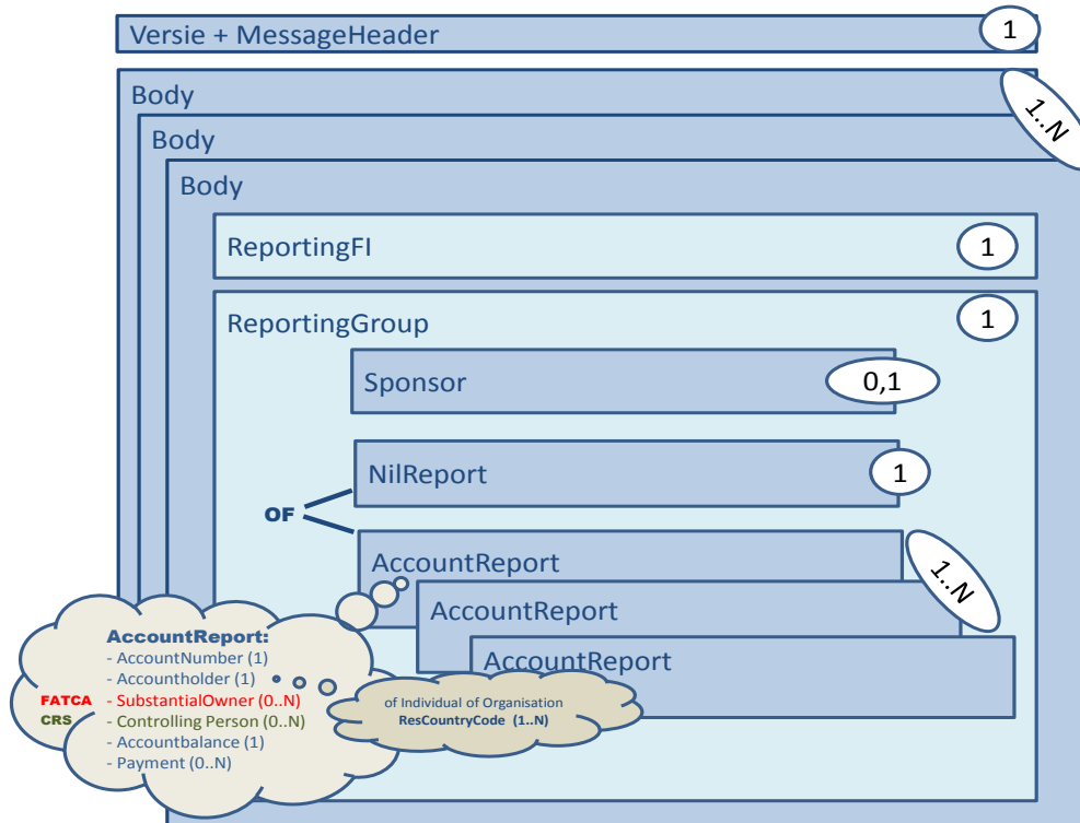
Figuur 3b: cardinaliteiten binnen het FATCA CRS XML berichtschema versie 2.0
