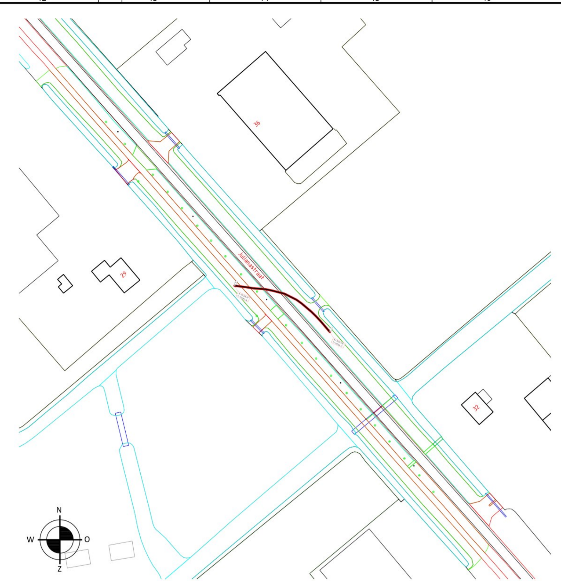
SITUATIE Schaal 1:1000
