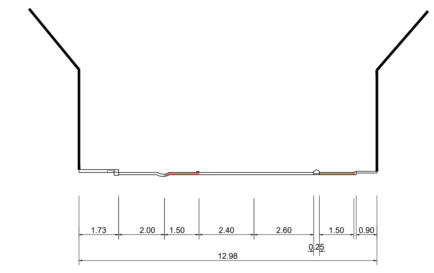
Dwarsprofiel
