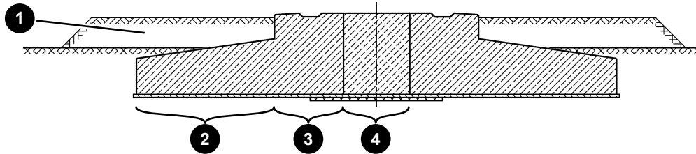
Abb. 1: Fundamentschnitt
