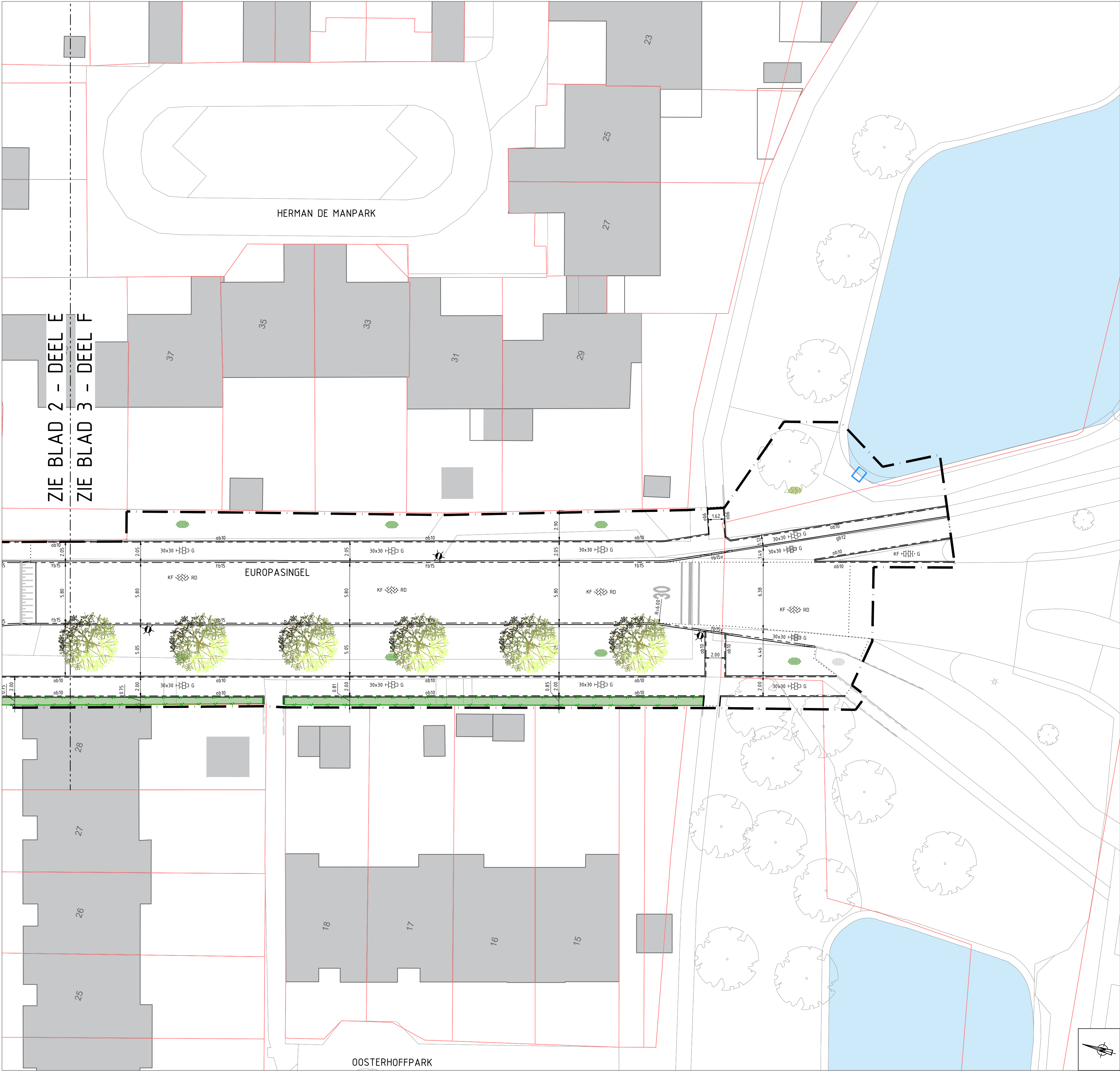
DEEL F SCHAAL 1:200
