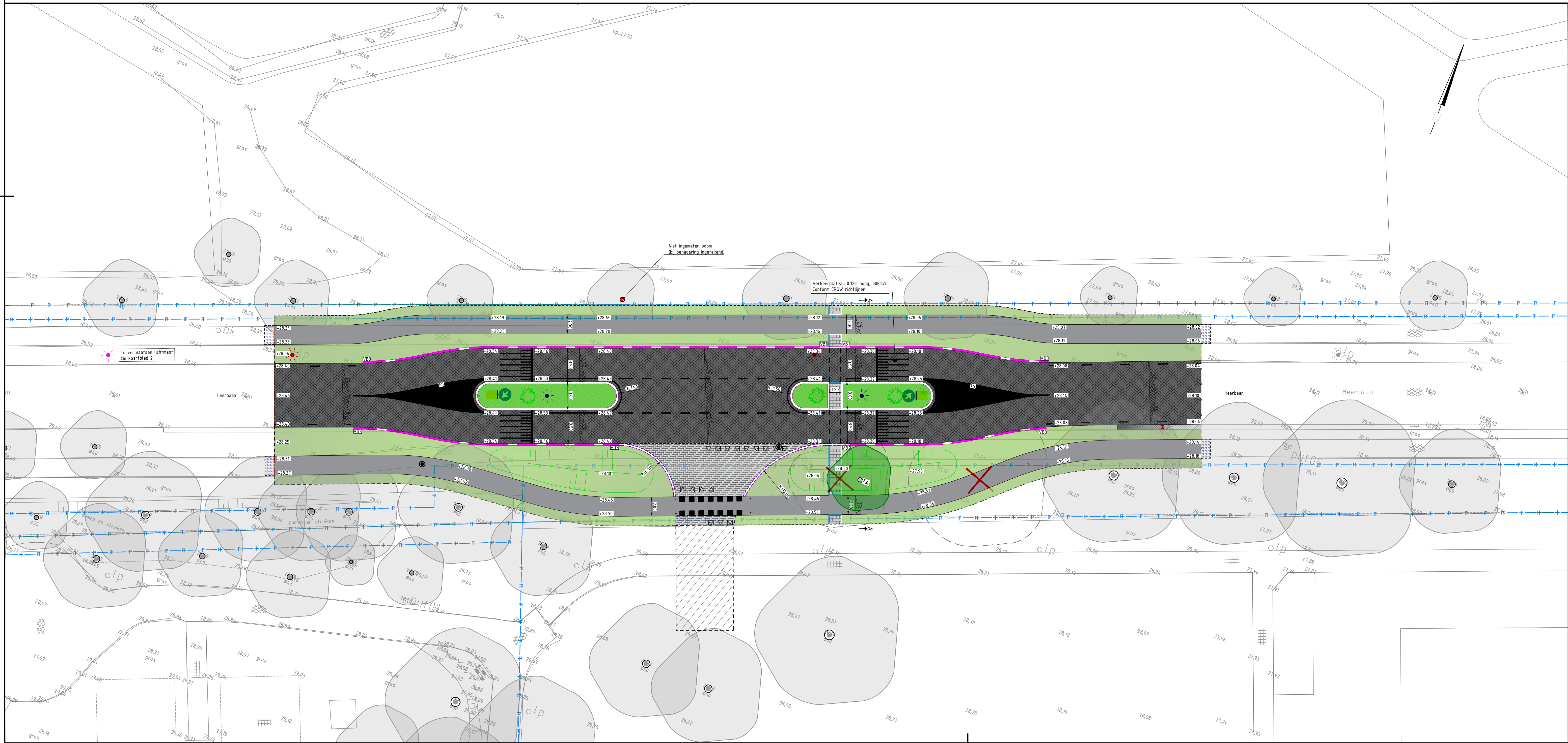
Principe detail 03: plateau (60km/uur) (12cm hoog) (bubeko) Schaal 120
