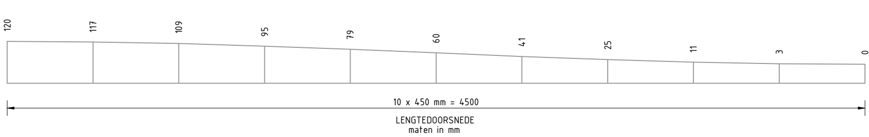
Principe detail 03: plateau (60km/uur) (12cm hoog) (bubeko) Schaal 120
