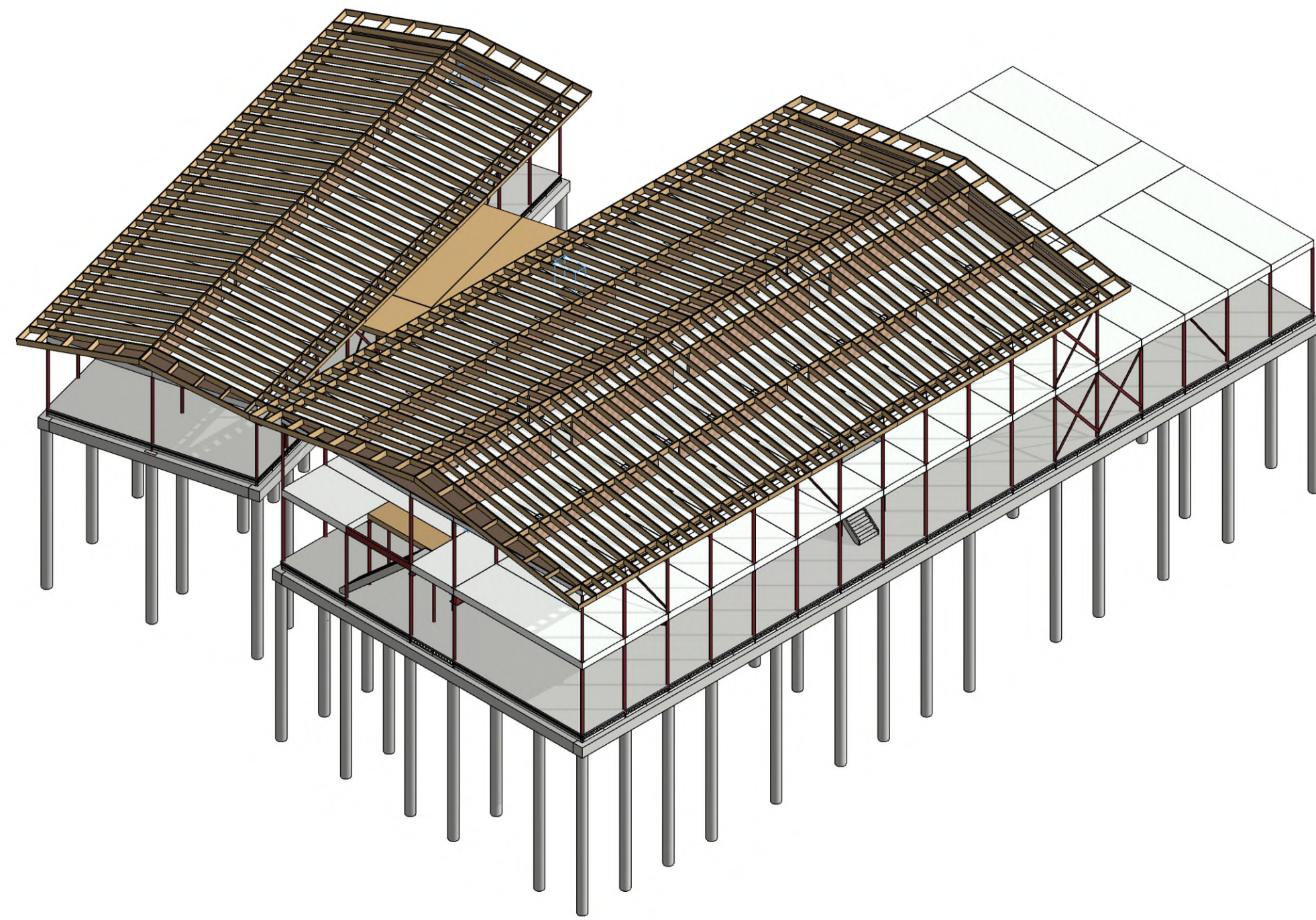
3D Constructie Zadeldaken
