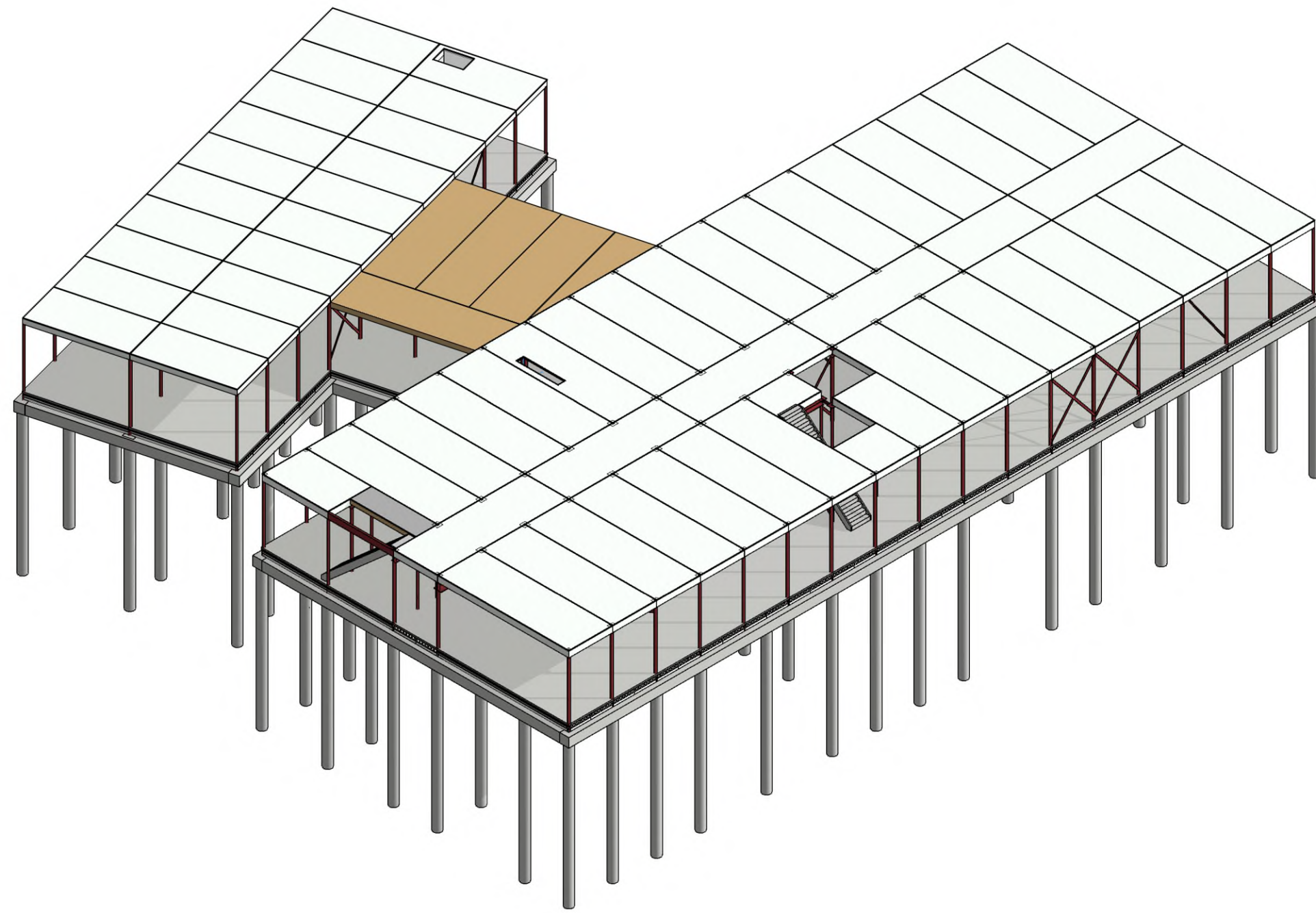
3D V1 Vloeren
