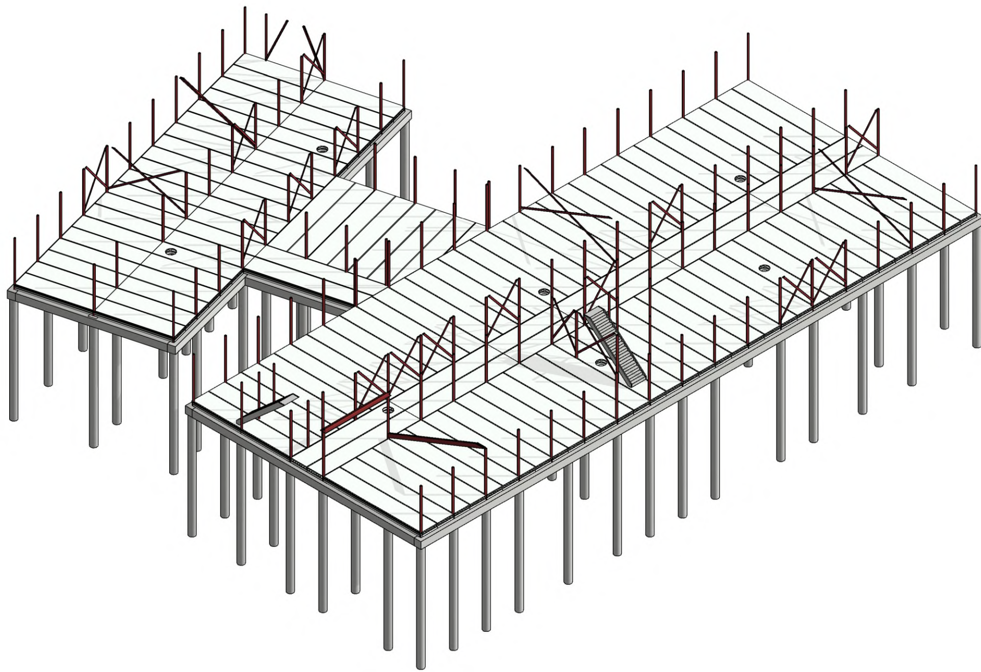
3D V0 Constructie en Vloeren
