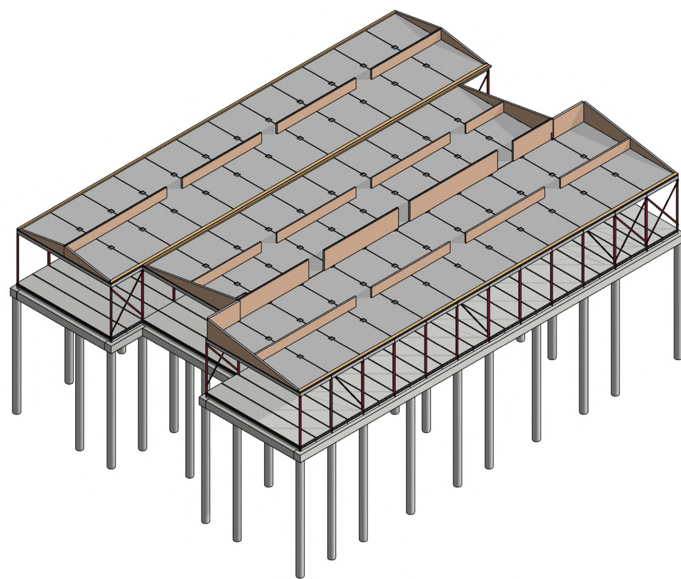
3D Constructie Zolder
