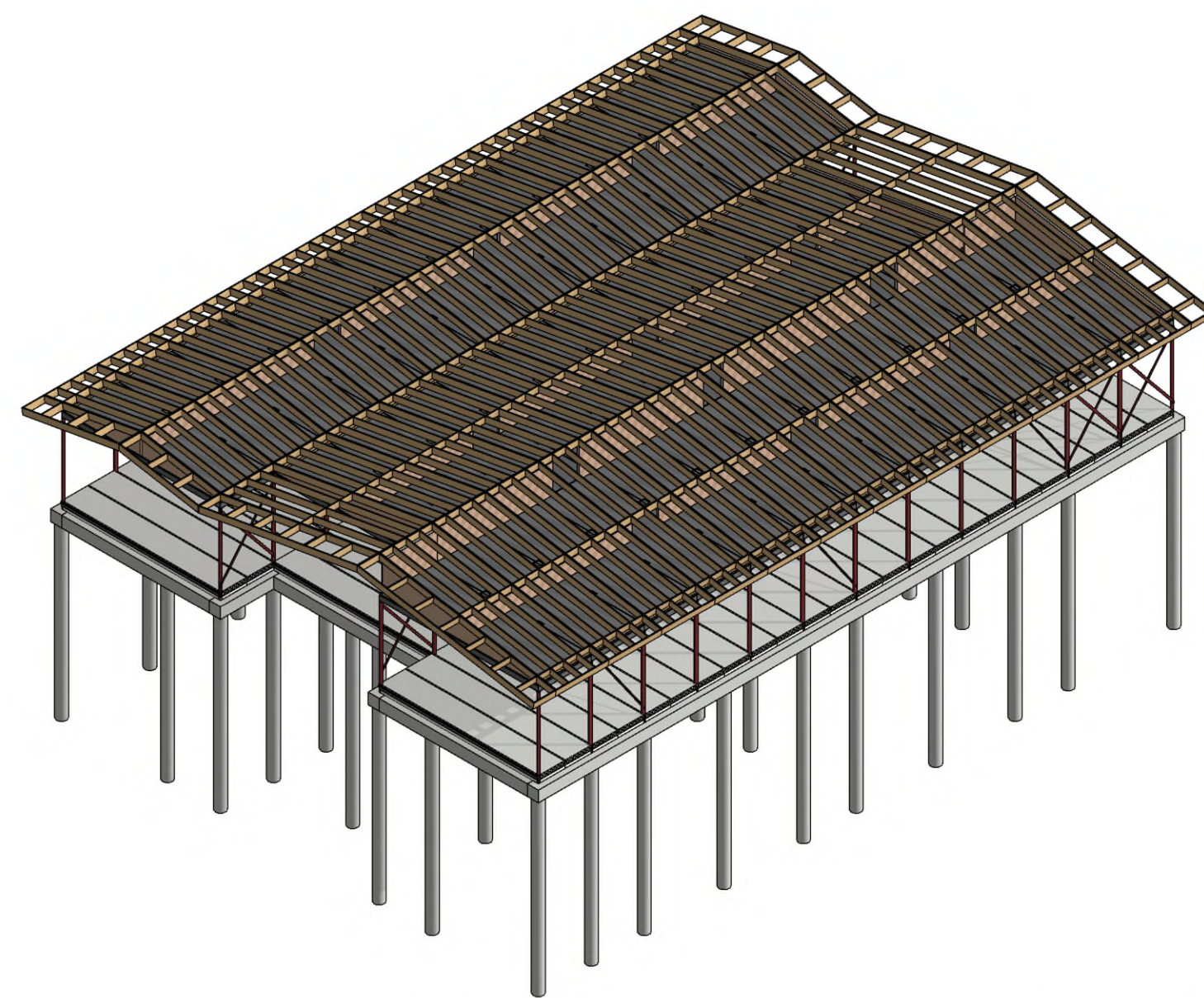
3D Constructie Zadeldak
