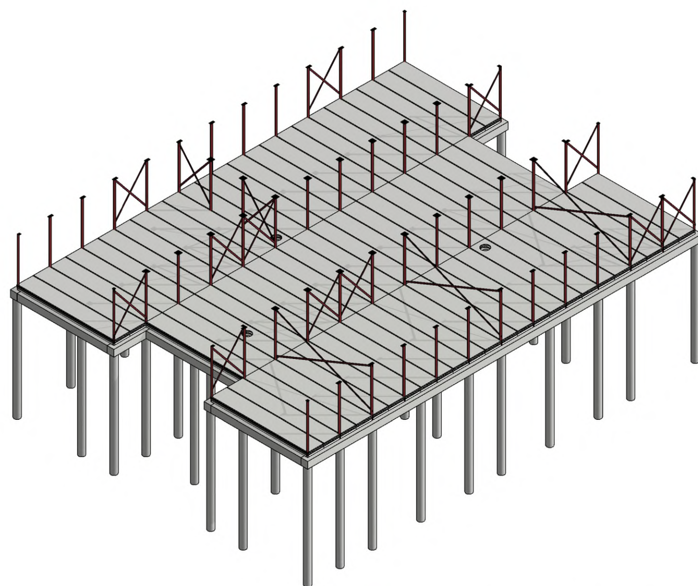
3D Draagconstructie
