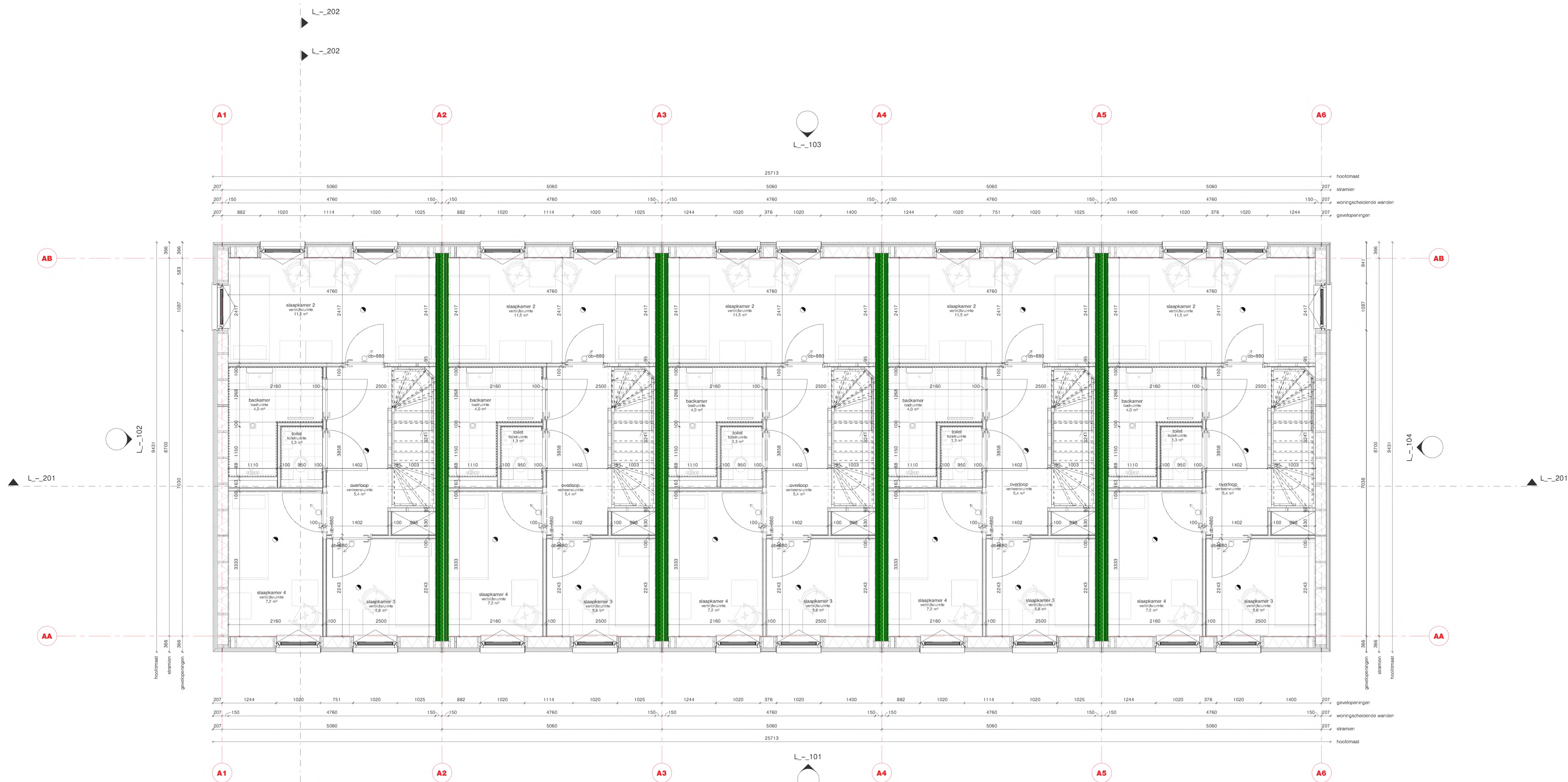
eerste verdieping (L_2_01) schaal: 1 : 50
