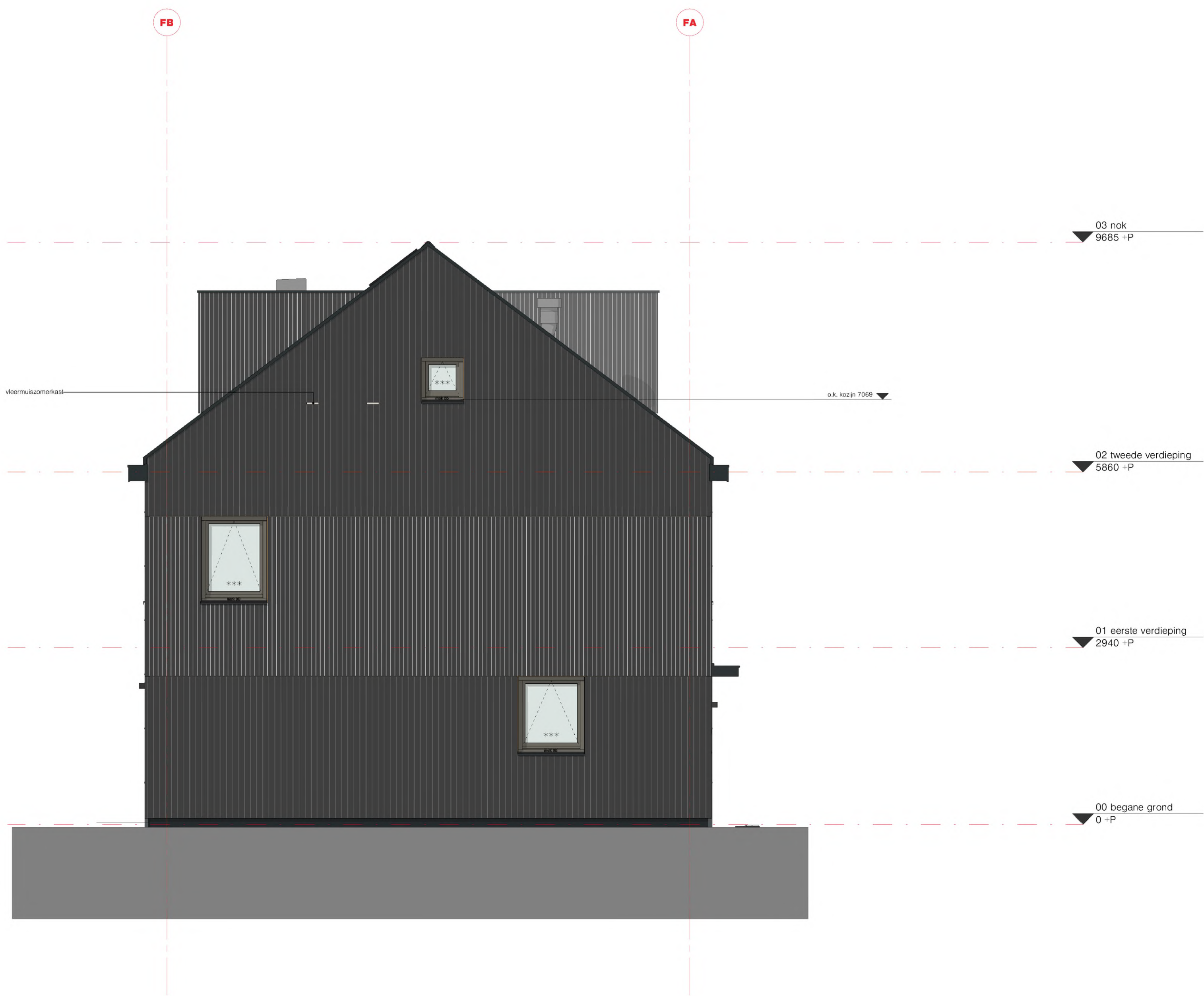
linker zijgevel (L_-_102) schaal: 1 : 50
