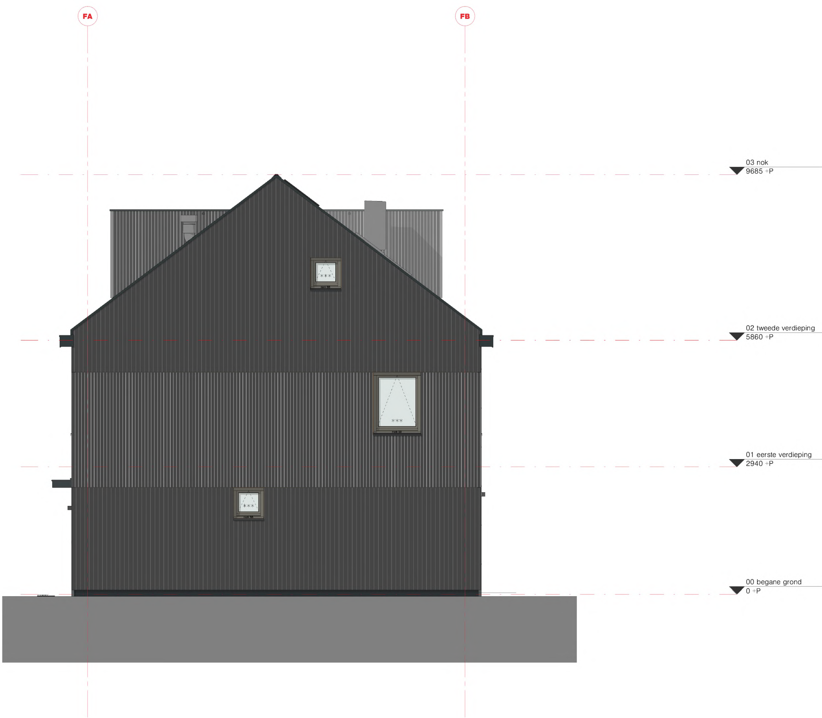
rechter zijgevel (L_-_104) schaal: 1 : 50
